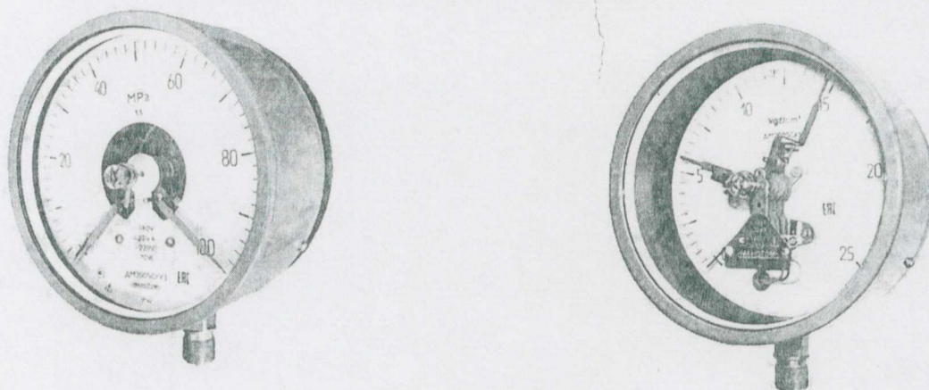
Рисунок 1 - Фотографии общего вида манометров, вакуумметров и мановакуумметров показывающих сигнализирующих ДМ2005Сг, ДВ2005Сг, ДА2005Сг
