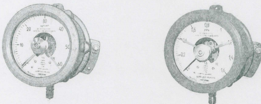
Рисунок 2 - Фотографии общего вида манометров, вакуумметров и мановакуумметров показывающих сигнализирующих ДМ2005Сг1Ех, ДВ2005Сг1Ех, ДА2005Сг1Ех
