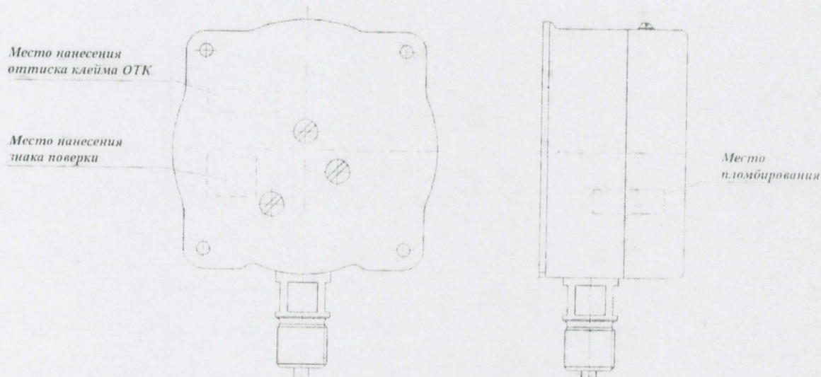
Рисунок 6 - Схема пломбирования от несанкционированного доступа и обозначение мест для нанесения оттисков клейма ОТК и знака поверки
