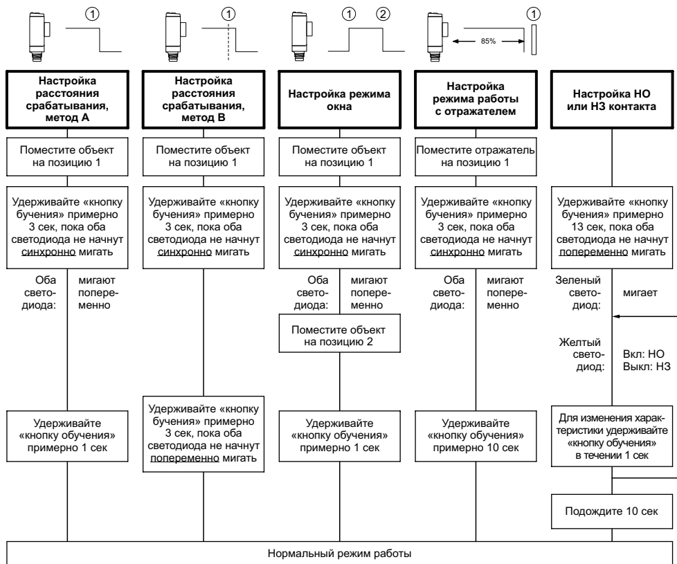
Рисунок 8 – Задание параметров с помощью процедуры «обучения» для датчика sks-15/CF
