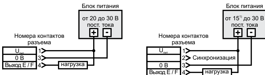
Рисунок 5 – Схема подключения датчиков sks-15/E , sks-15/CE и sks-15/CF (подключение по схеме с транзистором NPN)
