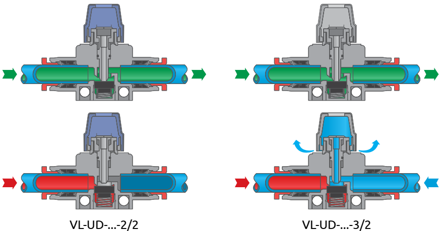
Рисунок 1 - Принцип действия фитинга
