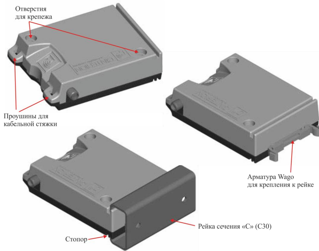
Рисунок 12: Монтаж BGS2T
