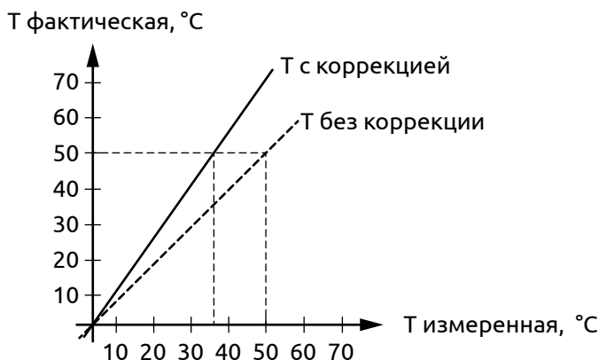
Рисунок 36 - Наклон характеристики измерительного входа
