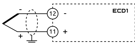
Рисунок 7 - Схема подключения термопар
