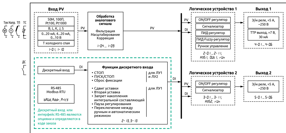
Рисунок 13 - Функциональная схема прибора
