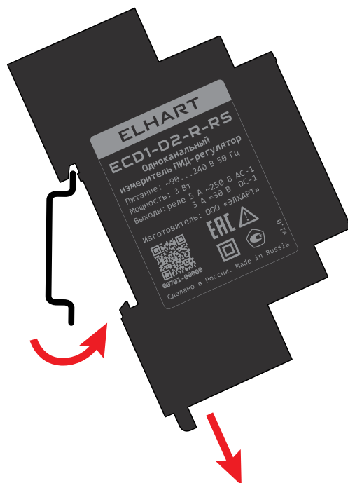
Рисунок 40 - Демонтаж прибора
