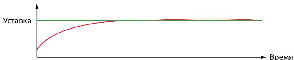
Рисунок 29 - Выход на уставку при избыточном значении дифференциальной составляющей
