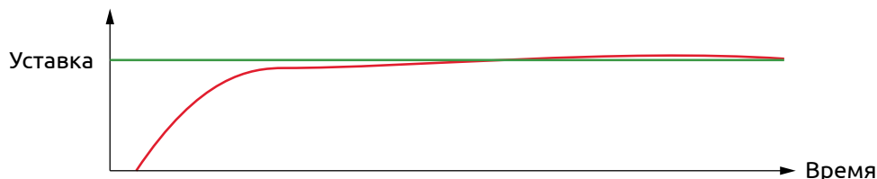
Рисунок 31 - Выход на уставку при недостаточном значении пропорциональной составляющей
