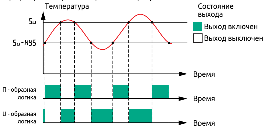
Рисунок 18 - Работа сигнализатора
