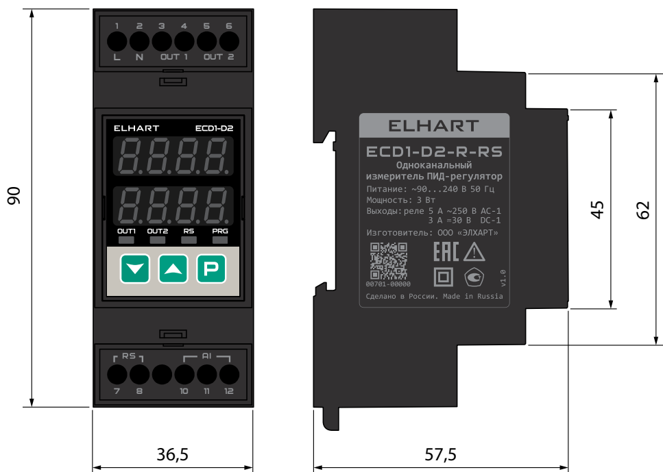
Рисунок 1 - Внешний вид и основные размеры прибора
