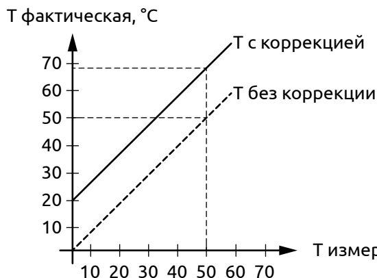
Рисунок 37 - Сдвиг характеристики измерительного входа
