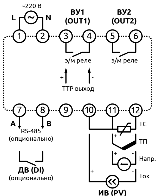
Рисунок 3 - Схема внешних соединений ECD1-D2
