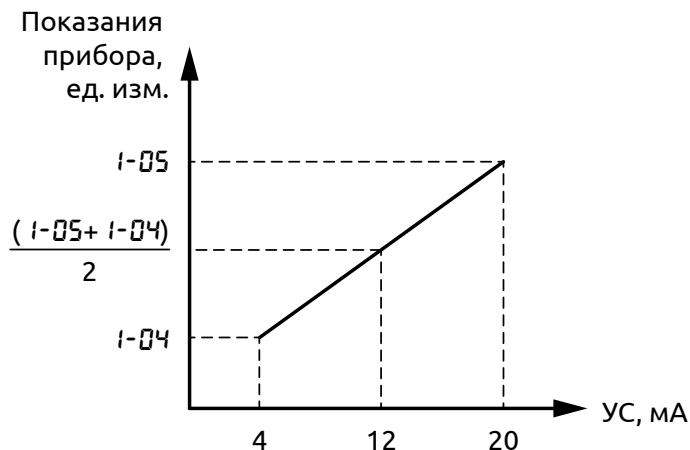
Рисунок 35 - Масштабирование диапазона датчиков с унифицированным сигналом 4...20 мА
