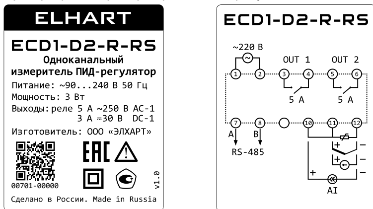
Рисунок 41 - Маркировка прибора
