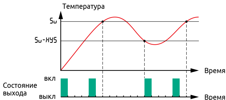
Рисунок 38 - Ограничение выходного сигнала двухпозиционного регулятора в режиме «нагреватель»
