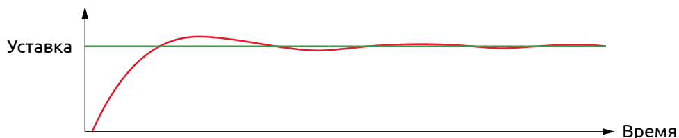
Рисунок 28 - Выход на уставку при недостаточном значении дифференциальной составляющей
