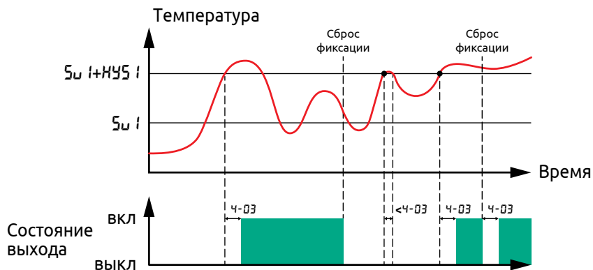
Рисунок 19 - Работа выхода при включенной фиксации
