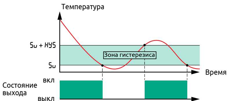
Рисунок 33 - Работа двухпозиционного регулятора в режиме «Холодильник»
