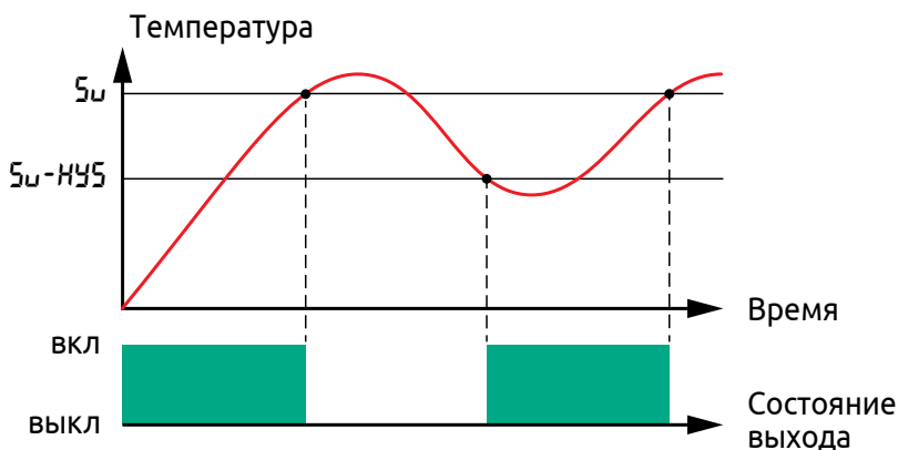
Рисунок 16 - Работа двухпозиционного регулятора в режиме «Нагреватель»
