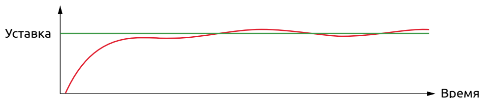
Рисунок 26 - Выход на уставку при избыточном значении интегральной составляющей и недостаточном значении смещения интегральной составляющей
