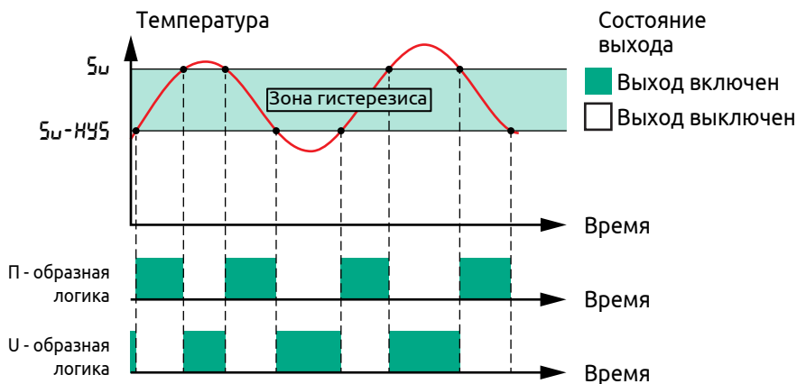
Рисунок 34 - Работа сигнализатора
