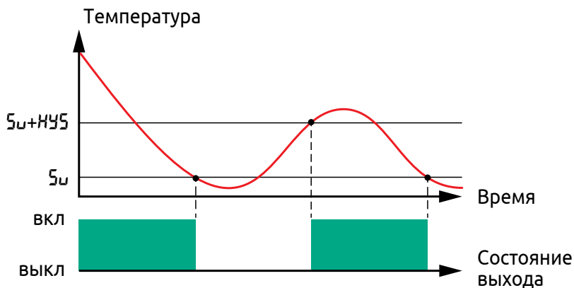
Рисунок 17 - Работа двухпозиционного регулятора в режиме «Холодильник»
