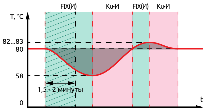
Рисунок 21 - График работы ПИД-Fuzzy-регулятора
