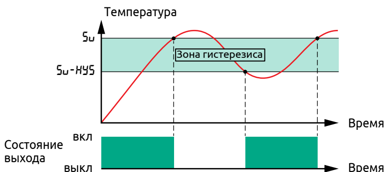
Рисунок 32 - Работа двухпозиционного регулятора в режиме «Нагреватель»
