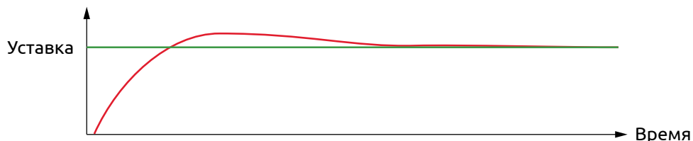
Рисунок 25 - Выход на уставку при избыточном значении смещения интегральной составляющей ПИД-регулятора
