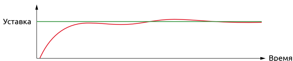
Рисунок 24 - Выход на уставку при недостаточном значении смещения интегральной составляющей ПИД-регулятора
