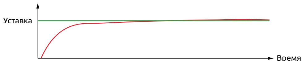
Рисунок 27 - Выход на уставку при недостаточном значении интегральной составляющей и недостаточном значении смещения интегральной составляющей
