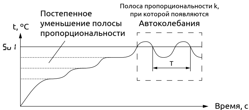
Рисунок 22 - Настройка ПИД-регулятора по методу Циглера-Никольса на примере регулирования температуры
