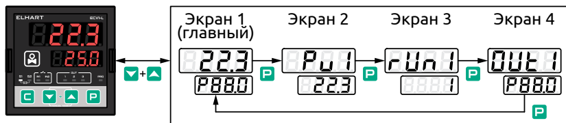
Рисунок 41 - Схема экранов для ручного управления выходом ЛУ1 «Нагреватель» и «Холодильник»
