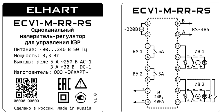
Рисунок 56 - Маркировка прибора
