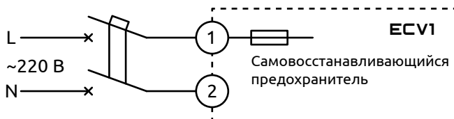
Рисунок 5 - Схема подключения напряжения питания к прибору
