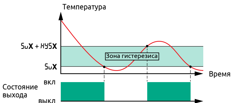
Рисунок 43 - Работа двухпозиционного регулятора в режиме «Холодильник»
