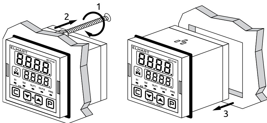
Рисунок 55 - Демонтаж прибора
