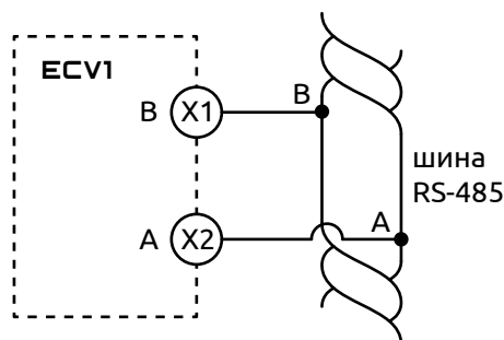
Рисунок 18 - Схема подключения RS-485
