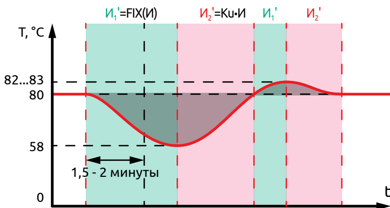
Рисунок 28 - График работы ПИД-Fuzzy-регулятора
