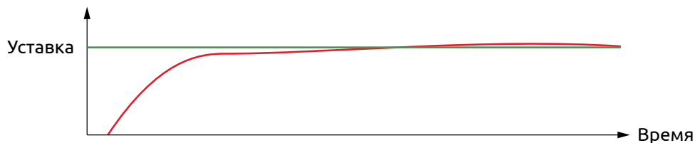
Рисунок 36 - Выход на уставку при недостаточном значении пропорциональной составляющей
