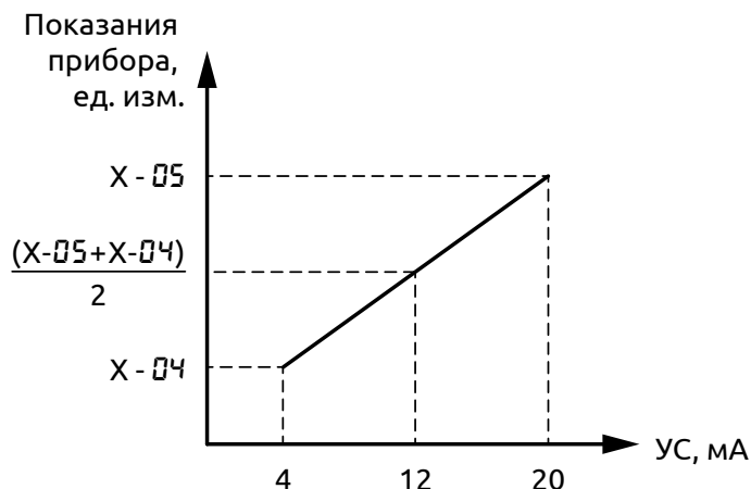
Рисунок 45 - Масштабирование диапазона датчиков с унифицированным сигналом 4...20 мА
