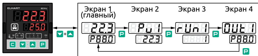
Рисунок 40 - Схема экранов для ручного управления выходом ЛУ1 «Нагреватель» или «Холодильник»
