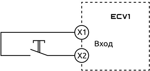
Рисунок 16 - Схема подключения кнопки «сухой контакт» к дискретному входу прибора
