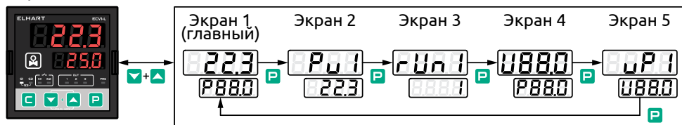
Рисунок 39 - Схема экранов для ручного управления КЗР
