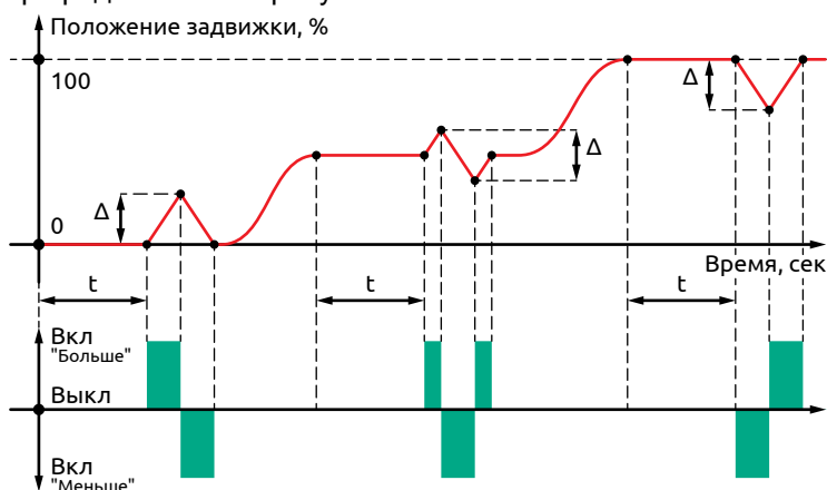
Рисунок 48 - Защита от замерзания
