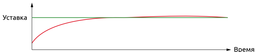
Рисунок 34 - Выход на уставку при избыточном значении дифференциальной составляющей
