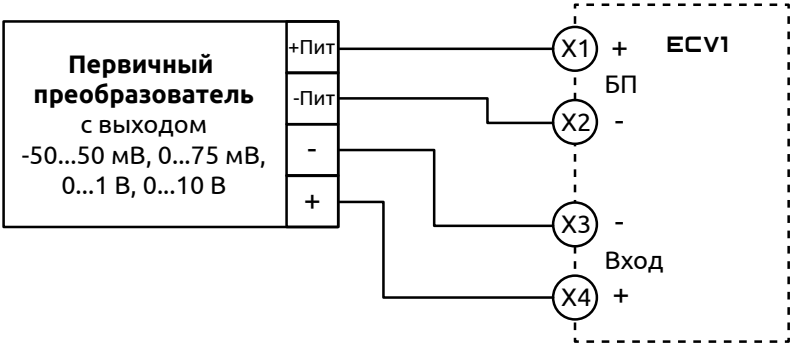
Рисунок 14 - Схема подключения первичного преобразователя с унифицированным сигналом напряжения с использованием встроенного блока питания
