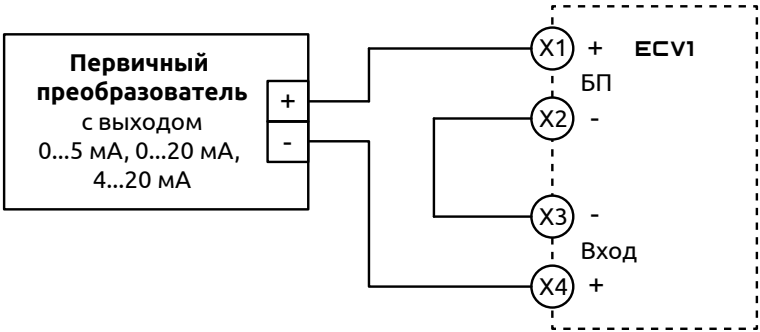
Рисунок 12 - Схема подключения первичного преобразователя с унифицированным сигналом тока к прибору с использованием встроенного в прибор блока питания
