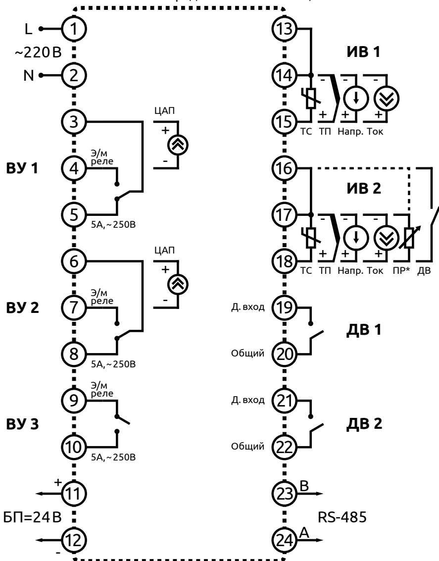
Рисунок 4 - Схема внешних соединений прибора ECV1-L
