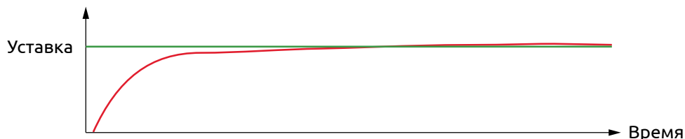
Рисунок 32 - Выход на уставку при недостаточном значении интегральной составляющей
