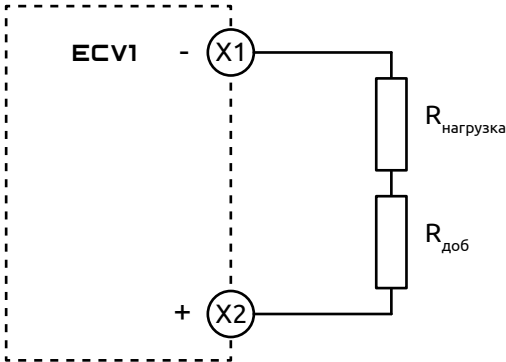
Рисунок 8 - Схема подключения нагрузки к выходу ЦАП прибора для получения унифицированного сигнала тока
