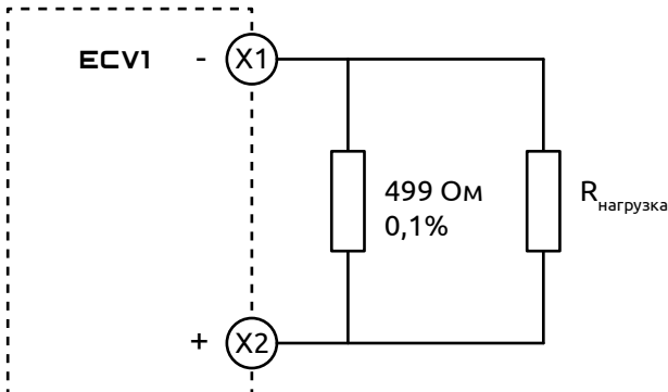
Рисунок 9 - Схема подключения нагрузки к выходу ЦАП прибора для получения унифицированного сигнала напряжения
