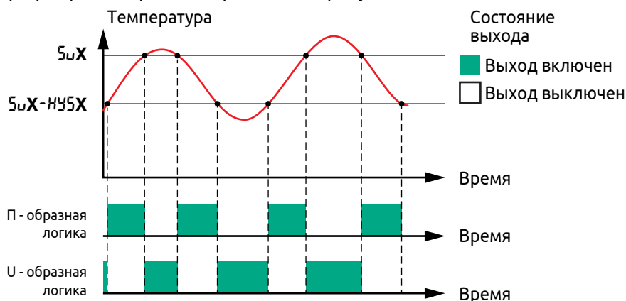
Рисунок 26 - Работа сигнализатора
