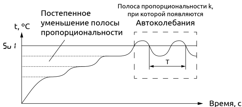
Рисунок 29 - Настройка ПИД-регулятора по методу Циглера-Никольса на примере регулирования температуры
