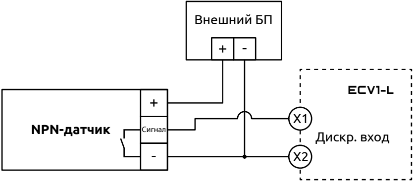
Рисунок 17 - Схема подключения NPN-датчиков к дискретным входам ECV1-L
