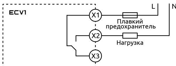
Рисунок 7 - Схема подключения нагрузки к выходному устройству э/м реле прибора ECV1-L
