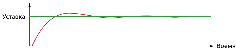
Рисунок 33 - Выход на уставку при недостаточном значении дифференциальной составляющей
