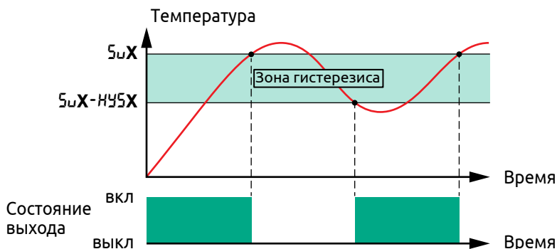
Рисунок 42 - Работа двухпозиционного регулятора в режиме «Нагреватель»
