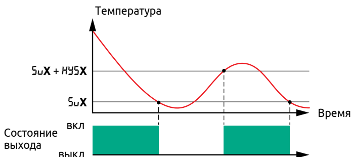
Рисунок 25 - Работа двухпозиционного регулятора в режиме «Холодильник»
