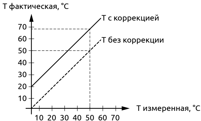
Рисунок 47 - Сдвиг характеристики измерительного входа
