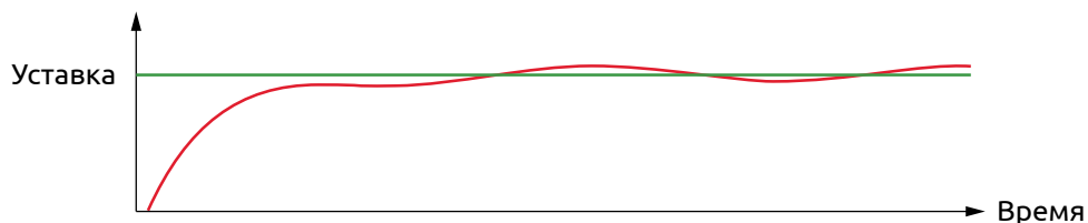
Рисунок 31 - Выход на уставку при избыточном значении интегральной составляющей
