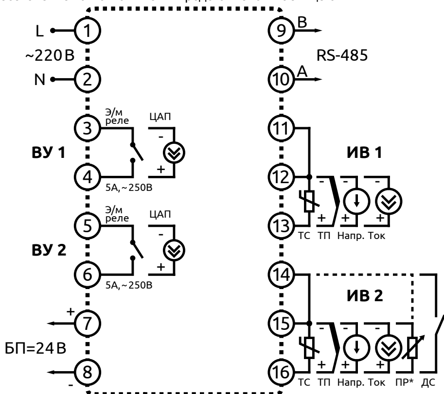
Рисунок 3 - Схема внешних соединений прибора ECV1-M
