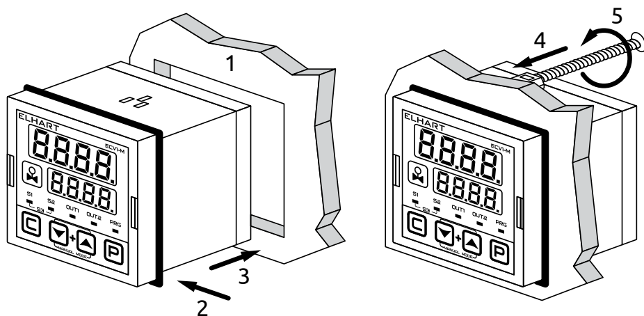
Рисунок 2 - Установка прибора в щит
