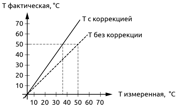
Рисунок 46 - Наклон характеристики измерительного входа
