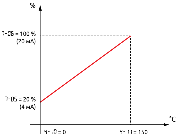
Рисунок 37 - Пример работы нормирующего преобразователя
