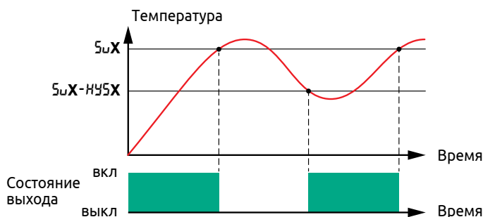
Рисунок 24 - Работа двухпозиционного регулятора в режиме «Нагреватель»
