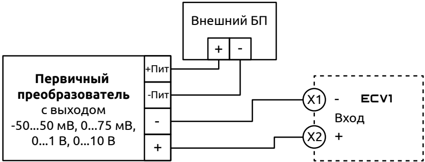
Рисунок 15 - Схема подключения первичного преобразователя с унифицированным сигналом напряжения с использованием внешнего блока питания
