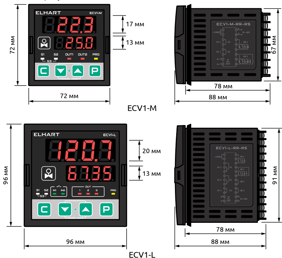
Рисунок 1 - Внешний вид и основные размеры прибора
