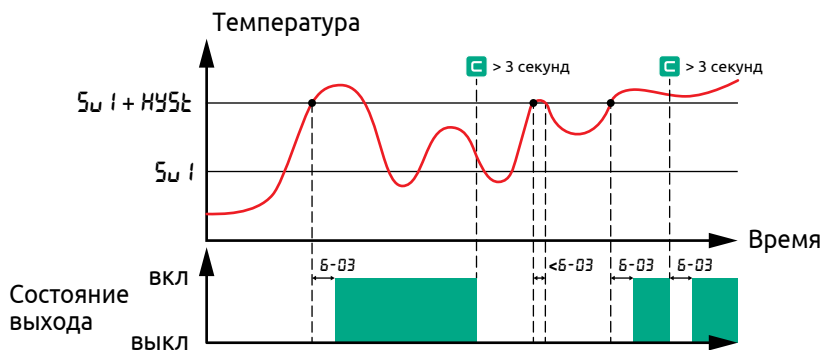
Рисунок 38 - Работа выхода при включенной фиксации
