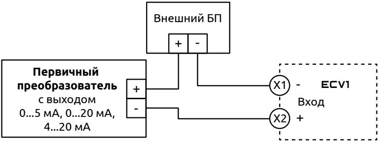
Рисунок 13 - Схема подключения первичного преобразователя с унифицированным сигналом тока к прибору с использованием внешнего блока питания
