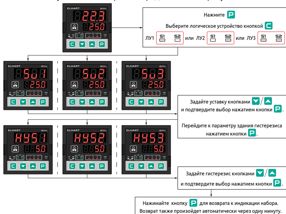
Рисунок 54 - Изменение уставки и гистерезиса
