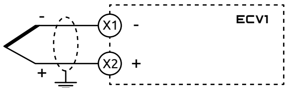
Рисунок 10 - Схема подключения термопары
