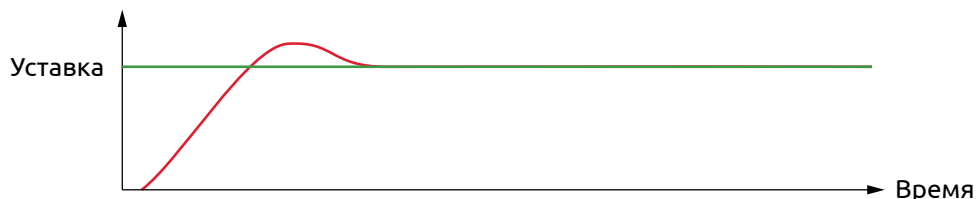
Рисунок 35 - Выход на уставку при избыточном значении пропорциональной составляющей
