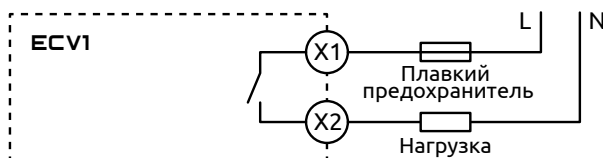
Рисунок 6 - Схема подключения нагрузки к выходному устройству э/м реле прибора ECV1-M (ВУЗ для ECV1-L)
