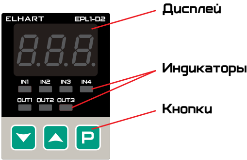
Рисунок 14 — Лицевая панель
