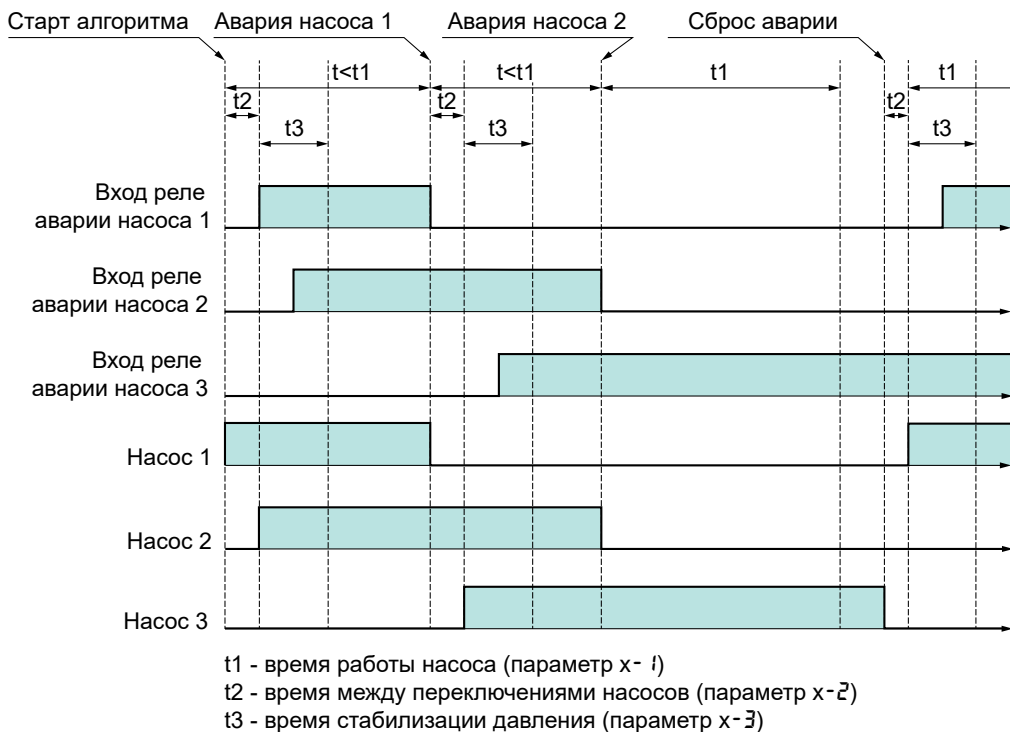
Рисунок 28 – Временная диаграмма АВР для схем 2+1 с двумя сломанными насосами
