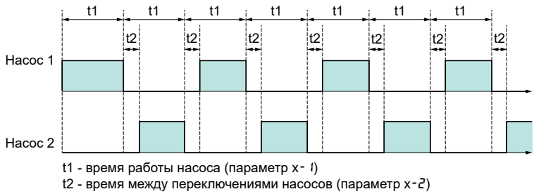
Рисунок 23 – Временная диаграмма смены насосов для схем 1+1
