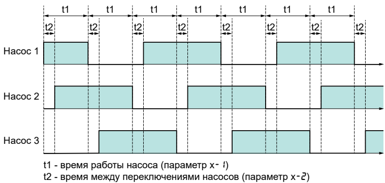
Рисунок 24 – Временная диаграмма смены насосов для схем 2+1
