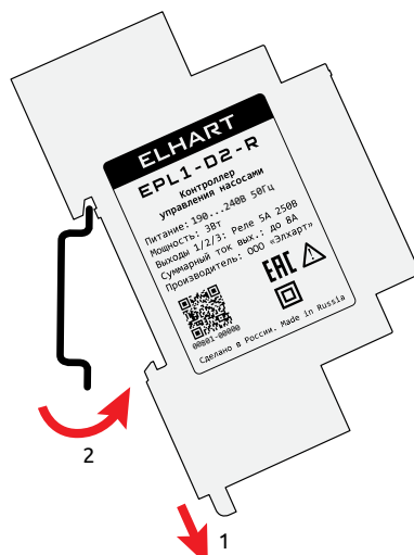
Рисунок 21 – Демонтаж прибора
