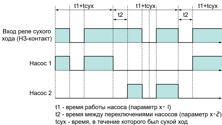
Рисунок 29 – Временная диаграмма АВР для схем 1+1 с "сухим ходом"
