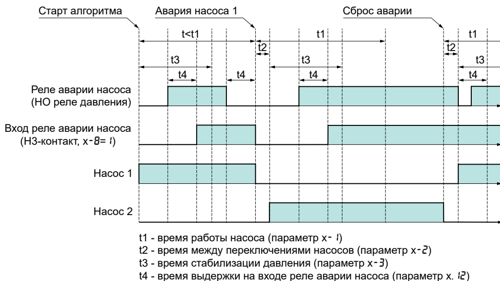
Рисунок 27 – Временная диаграмма АВР для схем 1+1 с одним сломанным насосом и сбросом аварии после истечения таймера работы насоса
