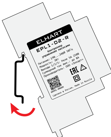
Рисунок 2 – Монтаж прибора
