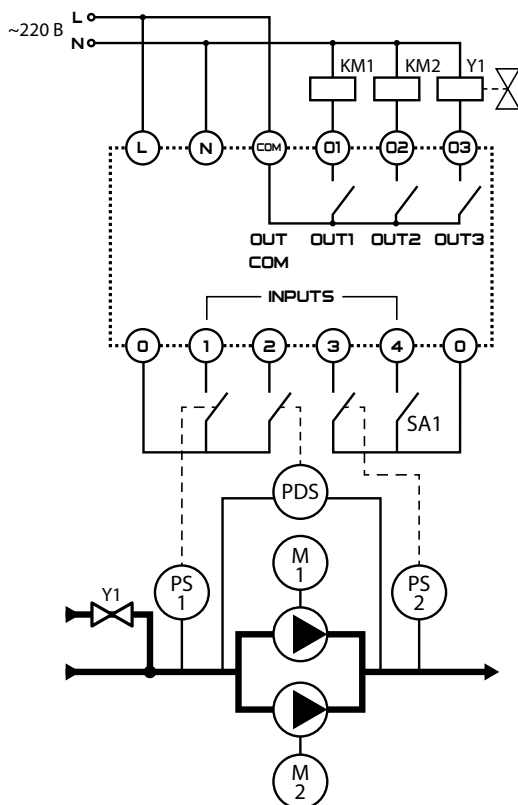
Рисунок 5 – Схема подключения для алгоритма 2 "Чередувание насосов по схеме 1+1 с АВР и подпиткой"
