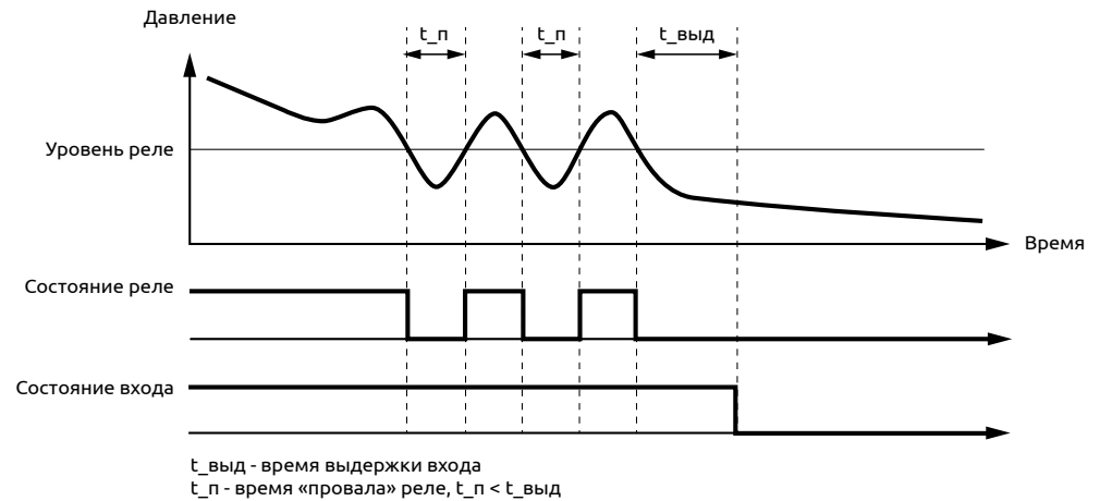
Рисунок 20 – Выдержка времени на входе
