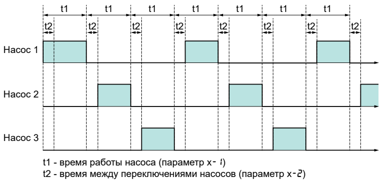
Рисунок 25 – Временная диаграмма смены насосов для схем 1+2
