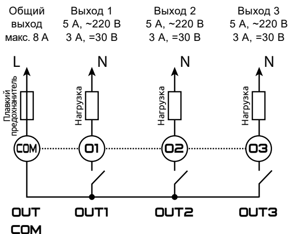
Рисунок 12 – Схема подключения выходов
