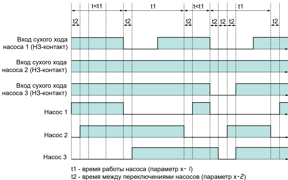
Рисунок 30 – Временная диаграмма АВР для схем с тремя насосами и датчиками "сухого хода" для каждого насоса
