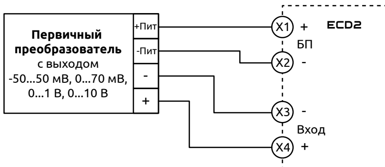
Рисунок 16 - Схема подключения первичного преобразователя с унифицированным сигналом напряжения с использованием встроенного блока питания
