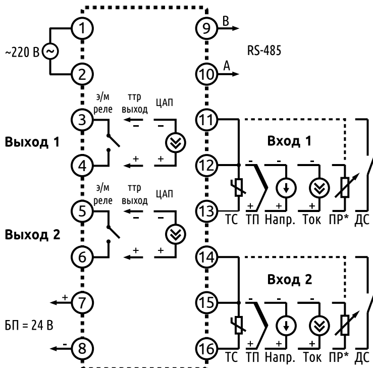
Рисунок 3 - Схема внешних соединений ECD2-M
