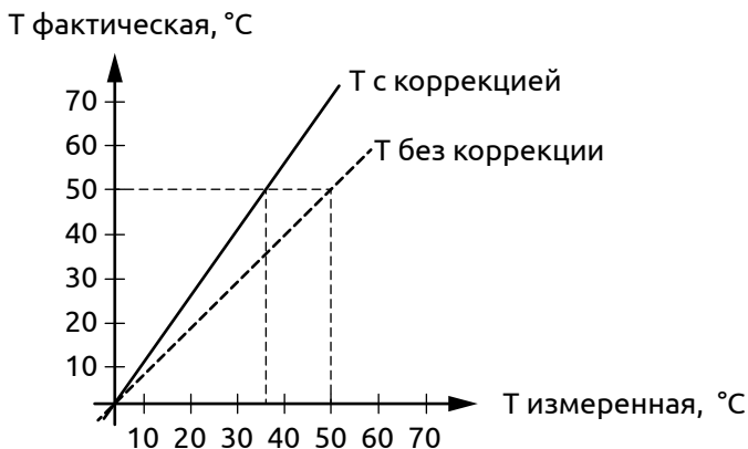
Рисунок 47 - Наклон характеристики измерительного входа
