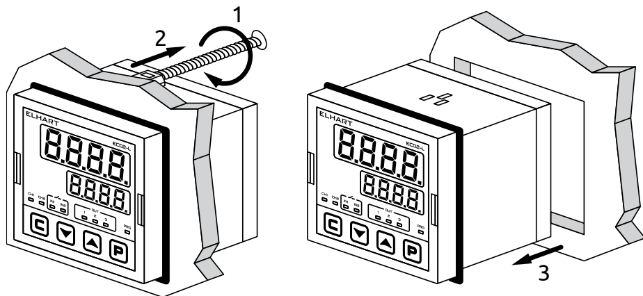
Рисунок 51 - Демонтаж прибора
