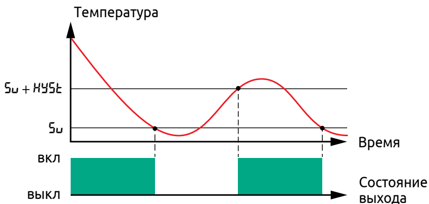
Рисунок 27 - Работа двухпозиционного регулятора в режиме «Холодильник»
