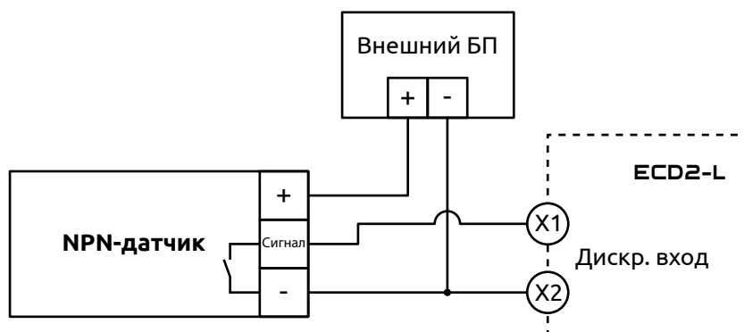
Рисунок 19 - Схема подключения NPN-датчиков к дискретным входам ECD2-L
