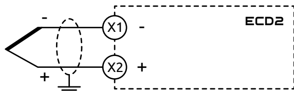
Рисунок 12 - Схема подключения термопар
