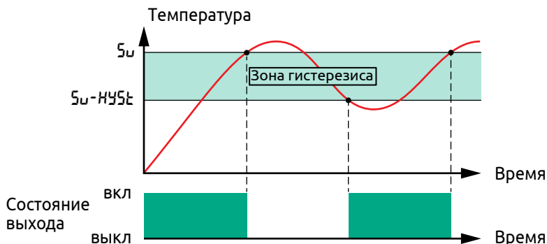
Рисунок 43 - Работа двухпозиционного регулятора в режиме «Нагреватель»
