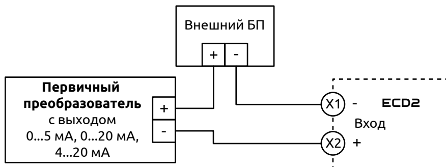
Рисунок 15 - Схема подключения первичного преобразователя с унифицированным сигналом тока с использованием внешнего блока питания
