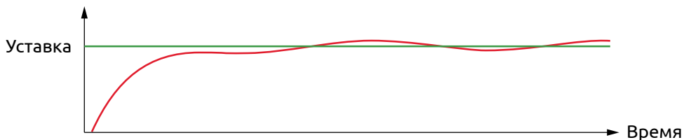
Рисунок 36 - Выход на уставку при избыточном значении интегральной составляющей и недостаточном значении смещения интегральной составляющей
