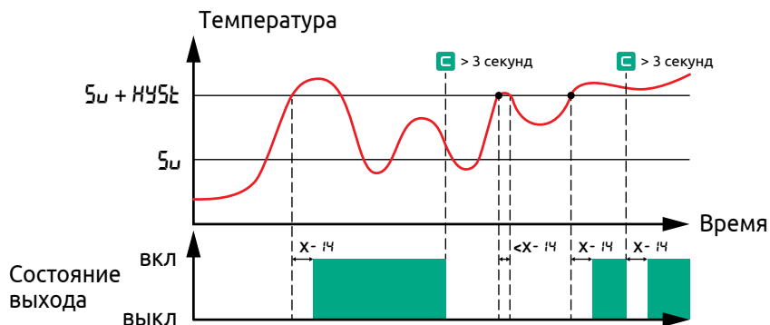
Рисунок 29 - Работа выхода при включенной фиксации
