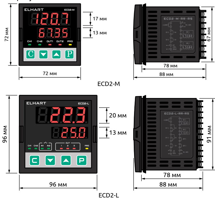
Рисунок 1 - Внешний вид и основные размеры прибора
