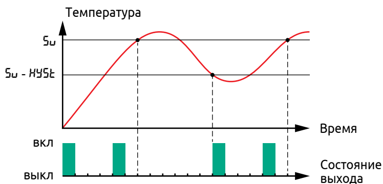
Рисунок 49 - Ограничение выходного сигнала двухпозиционного регулятора в режиме «нагреватель»
