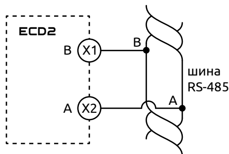
Рисунок 20 - Схема подключения RS-485
