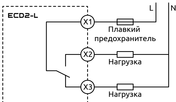
Рисунок 7 - Схема подключения нагрузки к выходу э/м реле прибора ECD2-L
