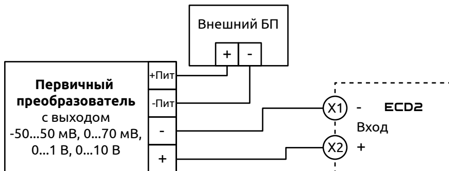
Рисунок 17 - Схема подключения первичного преобразователя с унифицированным сигналом напряжения и с использованием внешнего блока питания
