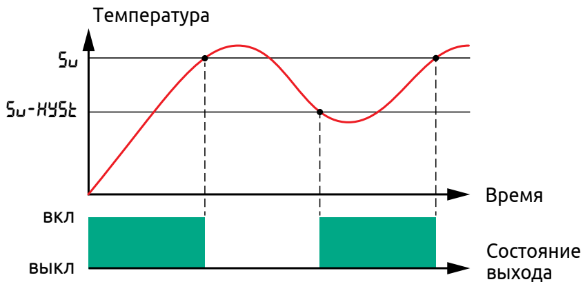
Рисунок 26 - Работа двухпозиционного регулятора в режиме «Нагреватель»
