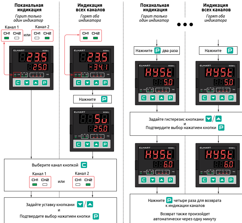
Рисунок 50 - Изменение уставки и гистерезиса
