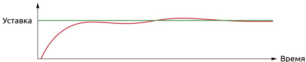
Рисунок 34 - Выход на уставку при недостаточном значении смещения интегральной составляющей ПИД-регулятора
