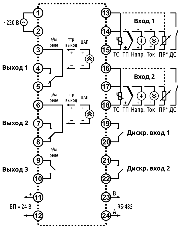
Рисунок 4 - Схема внешних соединений ECD2-L
