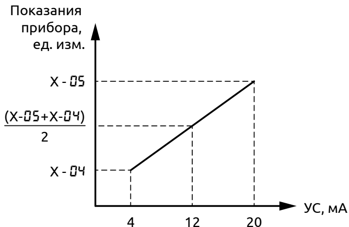
Рисунок 46 - Масштабирование диапазона датчиков с унифицированным сигналом 4...20 мА
