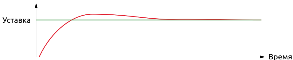
Рисунок 35 - Выход на уставку при избыточном значении смещения интегральной составляющей ПИД-регулятора
