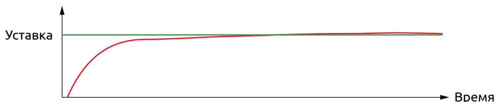
Рисунок 37 - Выход на уставку при недостаточном значении интегральной составляющей и недостаточном значении смещения интегральной составляющей
