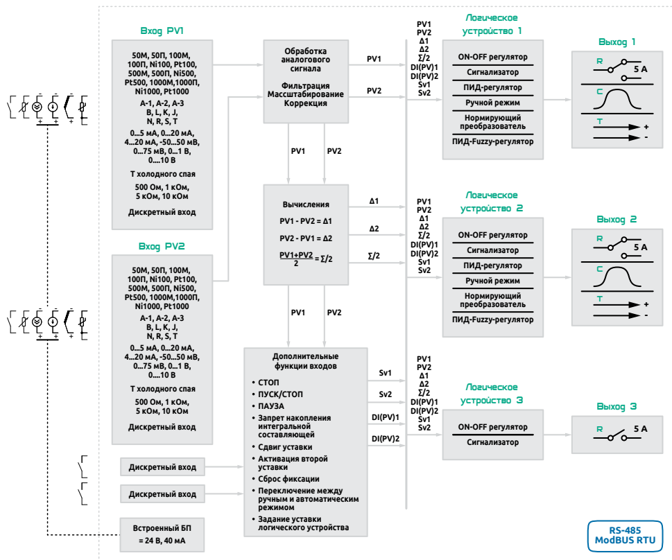
Рисунок 22 - Функциональная схема прибора ECD2-L
