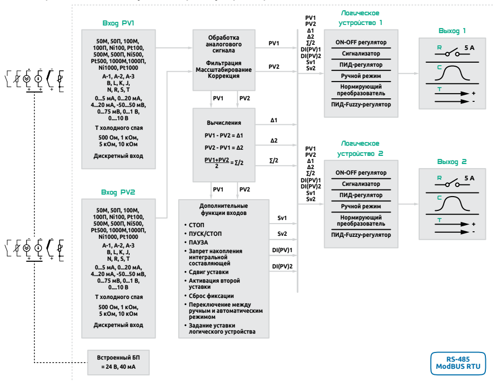
Рисунок 21 - Функциональная схема прибора ECD2-M
