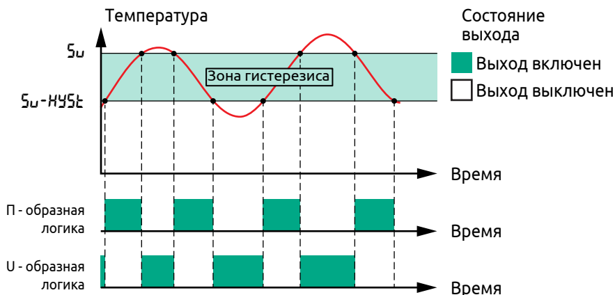
Рисунок 45 - Работа сигнализатора
