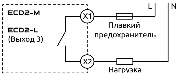
Рисунок 6 - Схема подключения нагрузки к выходу э/м реле прибора ECD2-M и к 3-му выходу прибора ECD2-L
