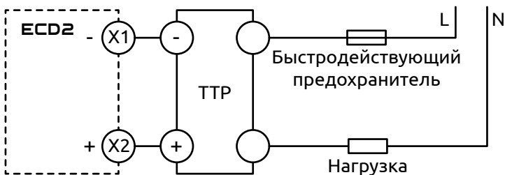
Рисунок 8 - Схема подключения твердотельного реле к ТТР выводу
