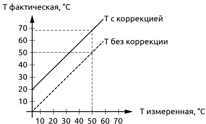
Рисунок 48 - Сдвиг характеристики измерительного входа
