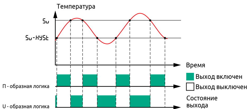
Рисунок 28 - Работа сигнализатора
