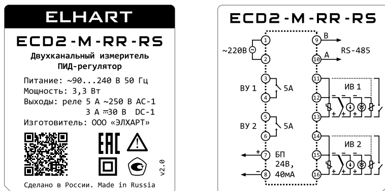
Рисунок 52 - Маркировка прибора
