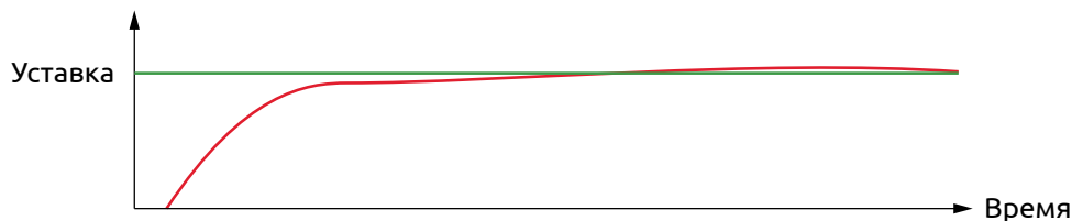
Рисунок 41 - Выход на уставку при недостаточном значении пропорциональной составляющей
