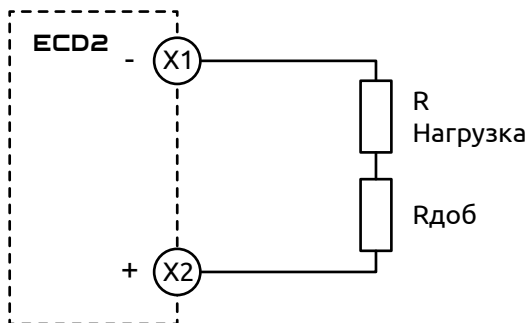
Рисунок 10 - Схема подключения нагрузки к выходу ЦАП прибора для получения унифицированного сигнала тока
