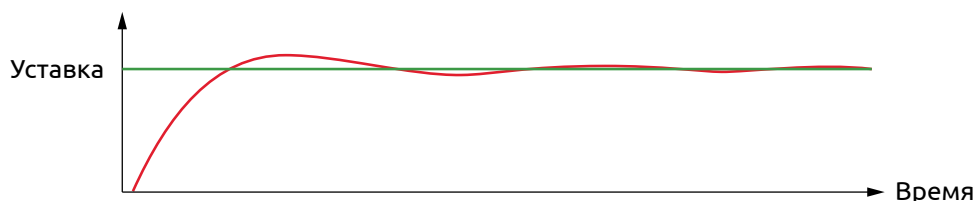
Рисунок 38 - Выход на уставку при недостаточном значении дифференциальной составляющей
