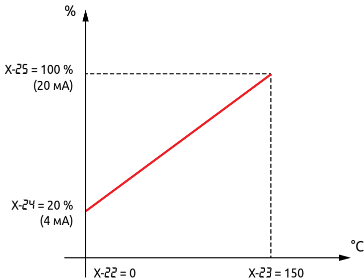
Рисунок 42 - Пример работы нормирующего преобразователя
