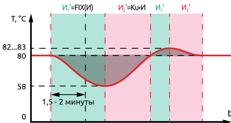
Рисунок 31 - График работы ПИД-Fuzzy-регулятора
