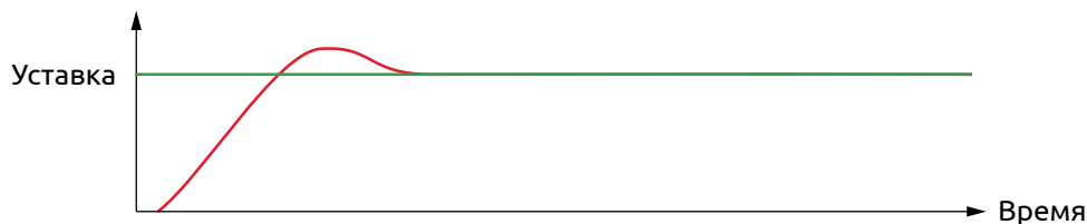
Рисунок 40 - Выход на уставку при избыточном значении пропорциональной составляющей
