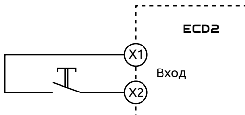
Рисунок 18 - Схема подключения кнопки «сухой контакт» к дискретному входу прибора
