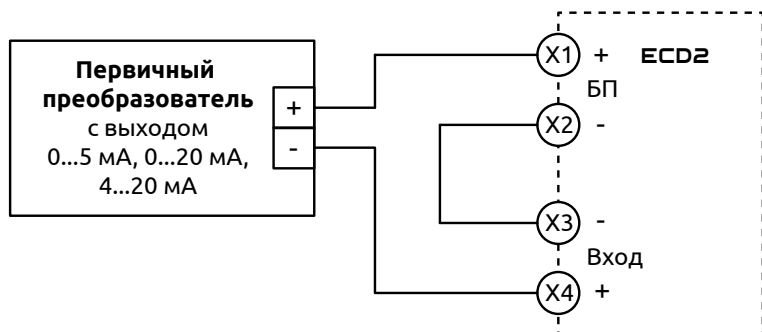
Рисунок 14 - Схема подключения первичного преобразователя с унифицированным сигналом тока с использованием встроенного блока питания
