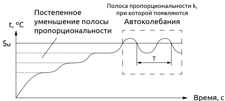
Рисунок 32 - Настройка ПИД-регулятора по методу Циглера-Никольса на примере регулирования температуры
