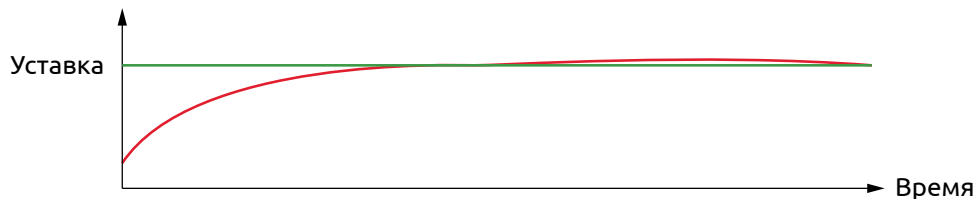
Рисунок 39 - Выход на уставку при избыточном значении дифференциальной составляющей
