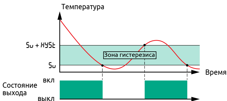
Рисунок 44 - Работа двухпозиционного регулятора в режиме «Холодильник»
