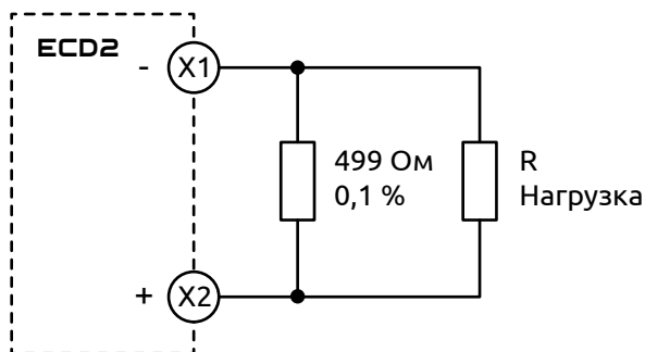
Рисунок 11 - Схема подключения нагрузки к выходу ЦАП прибора для получения унифицированного сигнала напряжения
