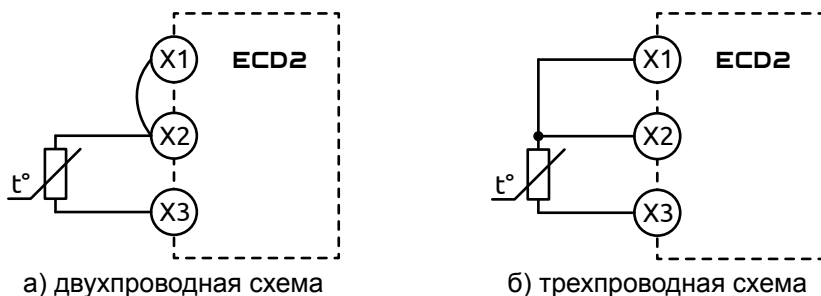
Рисунок 13 - Схема подключения термосопротивления
