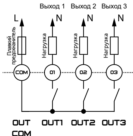
Рисунок 10 – Схема подключения выходов
