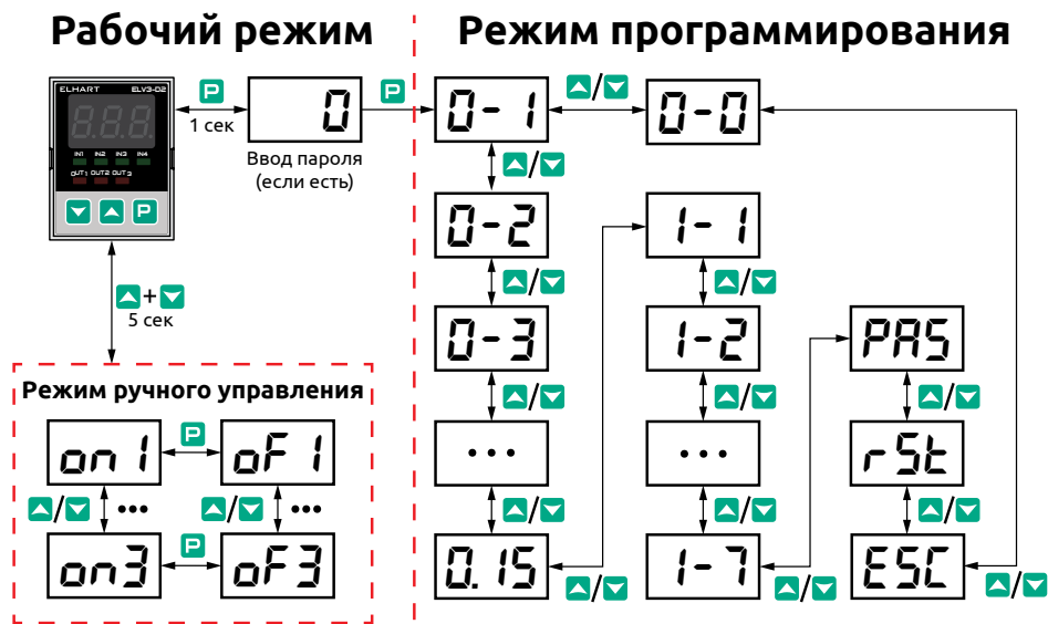
Рисунок 13 – Навигация в меню прибора
