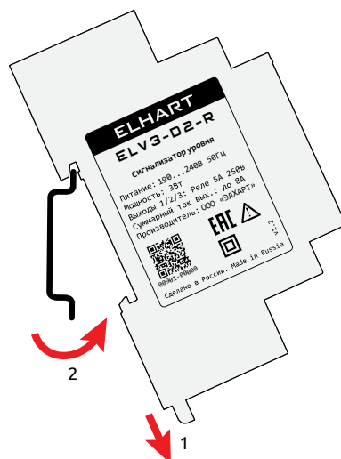
Рисунок 16 – Демонтаж прибора
