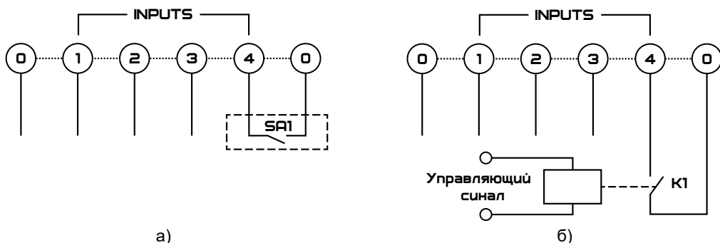
Рисунок 9 – Схема подключения входа блокировки
