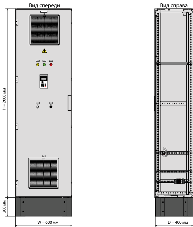
Рисунок 4.5 – Основные размеры ШУ серии КАСКАД 20М-xxx-1-К мощность 45, 55, 75, 90 кВт
