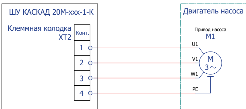
Рисунок 5.3 – Подключение двигателя насоса для модификаций ШУ КАСКАД 20М-xxx-1-К
