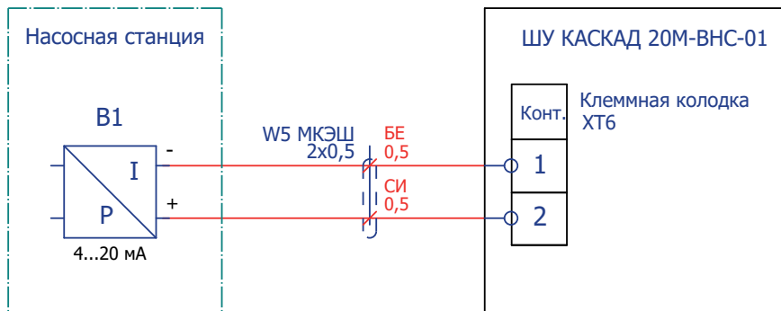
Рисунок 5.4 – Подключение датчика обратной связи на примере датчика давления
