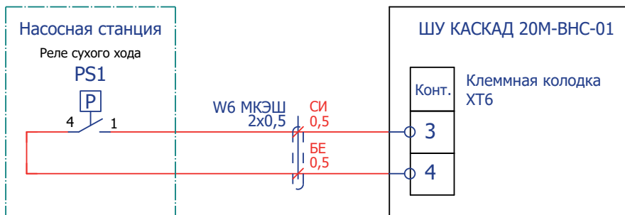
Рисунок 5.5 – Подключение реле сухого хода
