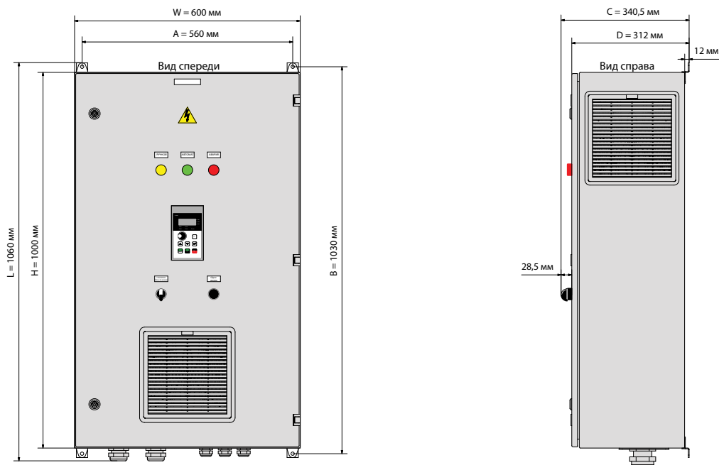
Рисунок 4.3 – Основные размеры ШУ серии КАСКАД 20М-xxx-1-К мощность 15 и 18,5 кВт
