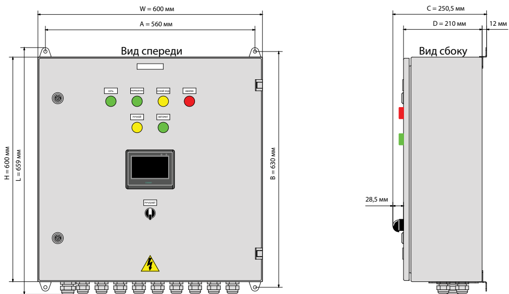
Рисунок 4.2 – Основные размеры ШУ серии КАСКАД 20М-ВНС-01
