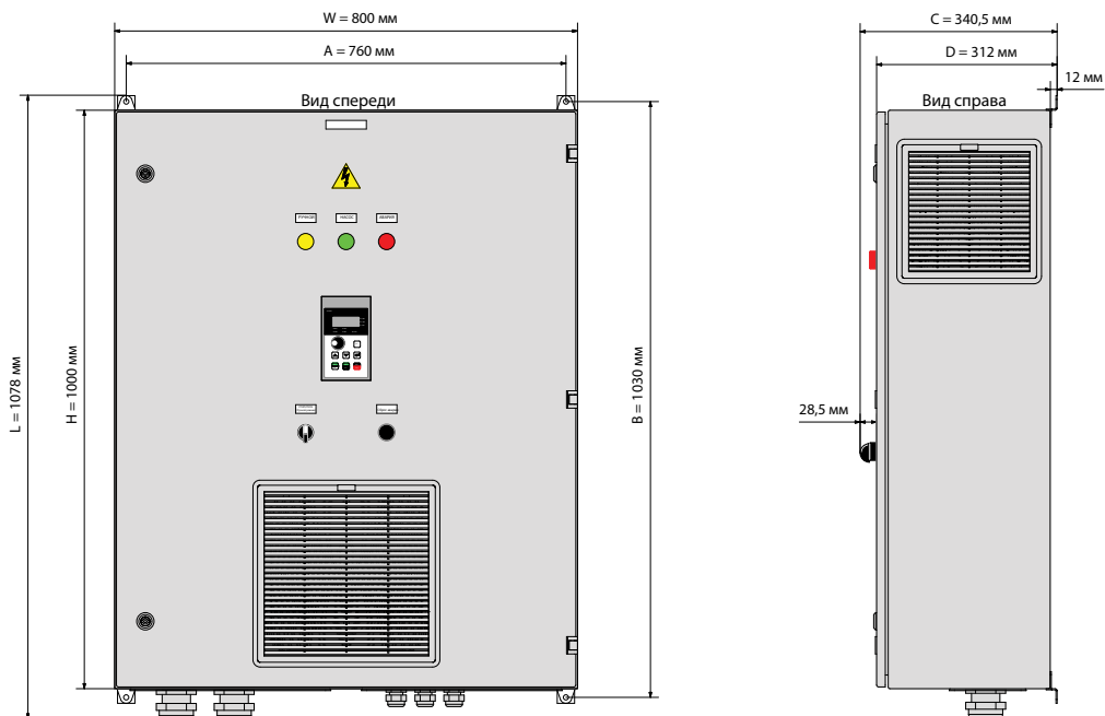
Рисунок 4.4 – Основные размеры ШУ серии КАСКАД 20М-xxx-1-К мощность 22, 30, 37 кВт
