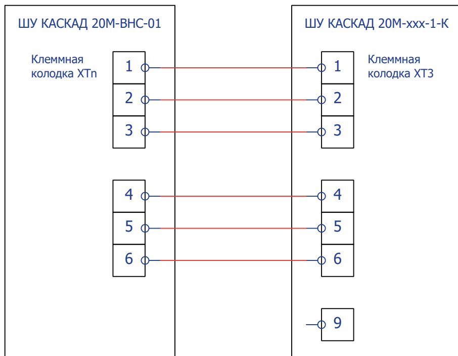
Рисунок 5.8 – Подключение шкафа «клиента» к шкафу «мастеру»
