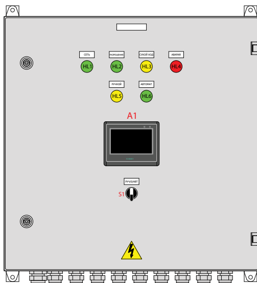
Рисунок 6.1 – Органы управления и индикации для модификаций ШУ КАСКАД 20М-ВНС-01
