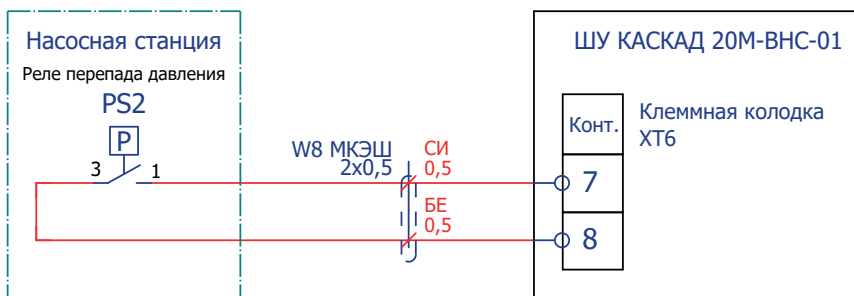
Рисунок 5.7 – Подключение реле перепада давления
