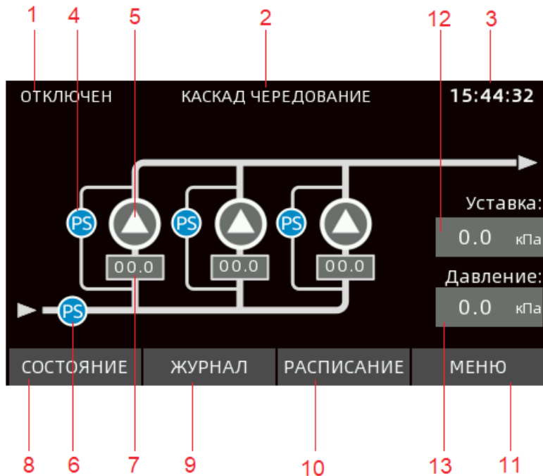
Рисунок 6.2 – Главный экран программы ШУ КАСКАД 20М
