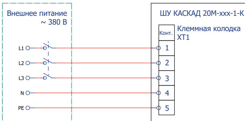
Рисунок 5.2 – Схема подключения питания для модификаций ШУ КАСКАД 20М-xxx-1-К
