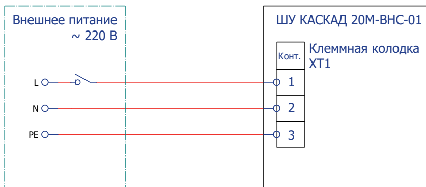
Рисунок 5.1 – Схема подключения питания для модификаций ШУ КАСКАД 20М-ВНС-01
