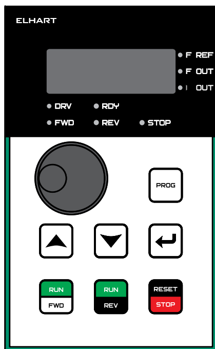
Рисунок 6.3 – Внешний вид пульта управления частотного преобразователя
