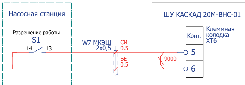
Рисунок 5.6 – Подключение сигнала разрешения работы
