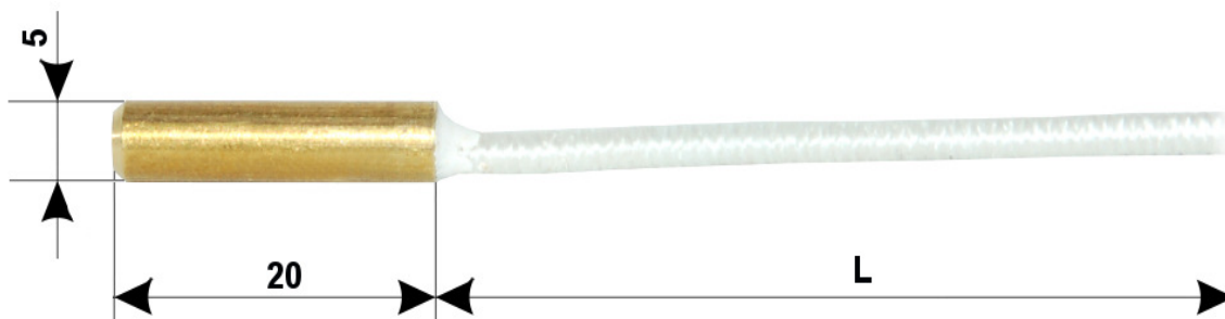
Рис.1 — Датчик температуры ДТПЛ014
