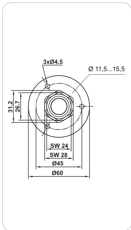
Тип ZA 24 для монтажа в воздуховодах
