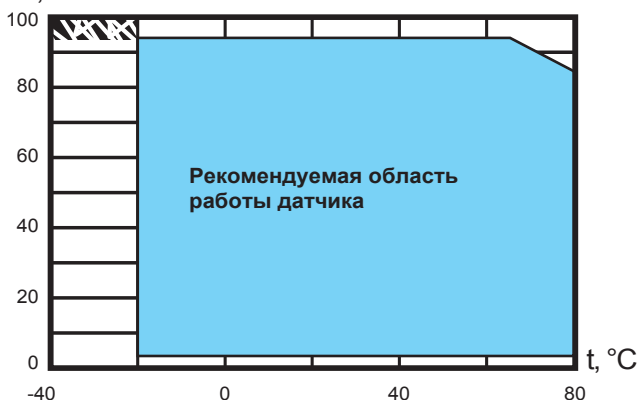
Диаграмма 1. Допустимые температурно-влажностные характеристики
