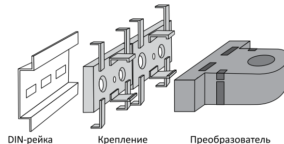
Рисунок 3 – Монтаж преобразователя на DIN-рейку
