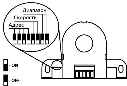
Рисунок 5 – Расположение DIP переключателей
