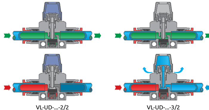
Рисунок 1 – Принцип действия фитинга
