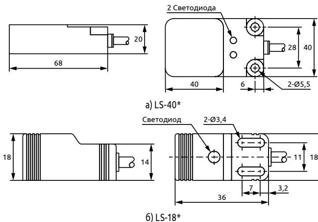
Рисунок 2 – Габаритные размеры
