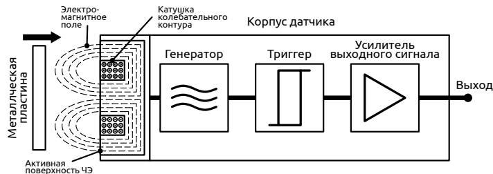
Рисунок 1 – Структура бесконтактного индуктивного датчика
