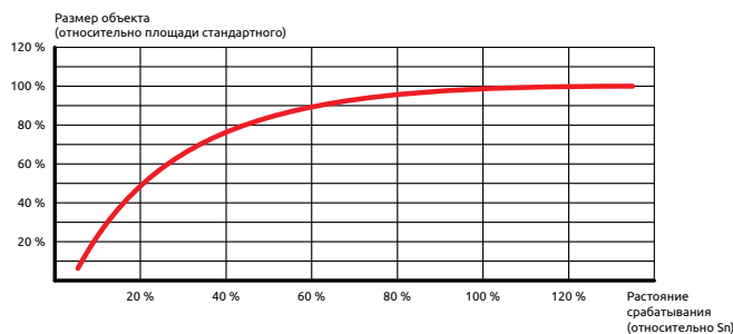
Рисунок 5 – Зависимость номинального рабочего диапазона от размера объекта воздействия
