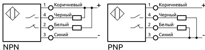
Рисунок 4 – Схема подключения индуктивных датчиков
