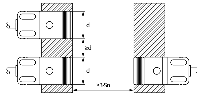
Рисунок 3 – Способы установки датчиков в металл
