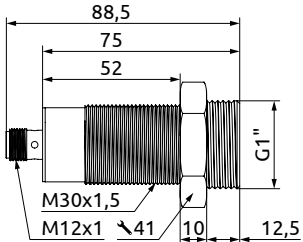
Рисунок 1 - UCS.*1-250-**-**, мм
