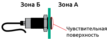
Рисунок 2 — Давление со стороны чувствительной поверхности
