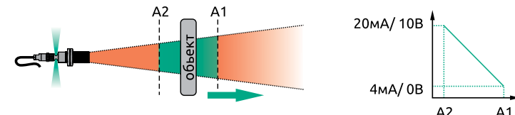
Рисунок 19 – Спадающий выходной сигнал
