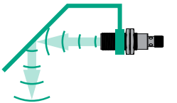
Рисунок 7 — Применение отражателя
