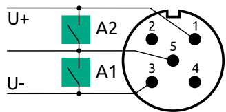
Рисунок 10 – Вход teach-in
