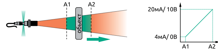
Рисунок 18 – Нарастающий выходной сигнал
