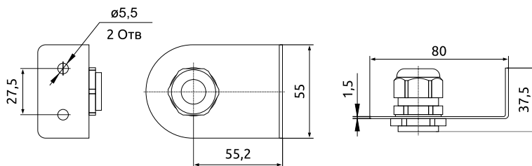
Рисунок 2 - Габаритные размеры консоли НТЕ-HoldW
