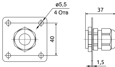
Рисунок 1 - Габаритные размеры консоли НТЕ-HoldC
