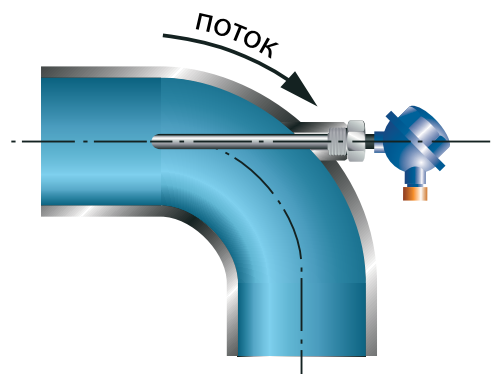
Рисунок 6 - Монтаж в колено трубы
