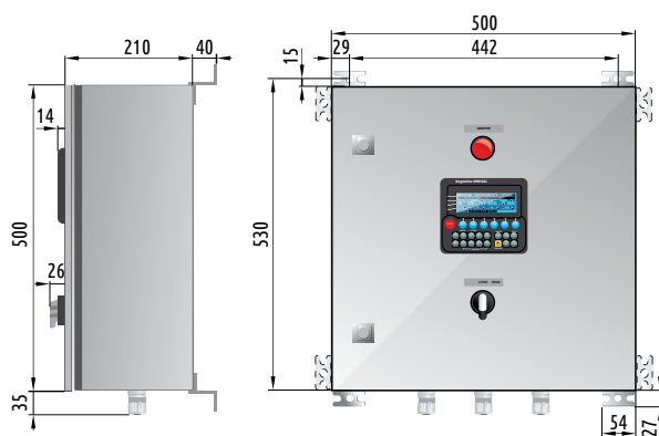
Шкаф управления КОНТУР-С1 500×500×210 мм
