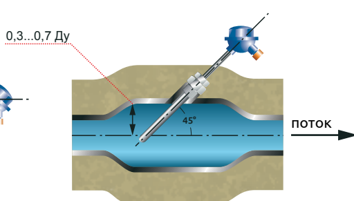
Рисунок 4 - Монтаж в расширение для узких участков трубопровода
