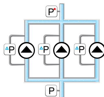
КАСКАД 101 xxx-3-x Управление тремя насосами
