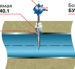
Рисунок 1 - Прямой монтаж
