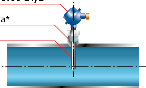
Рисунок 5 - Прямой монтаж
