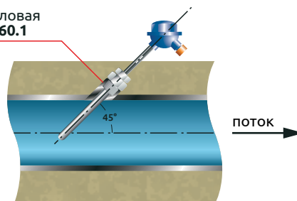
Рисунок 2 - Монтаж под углом 45°
