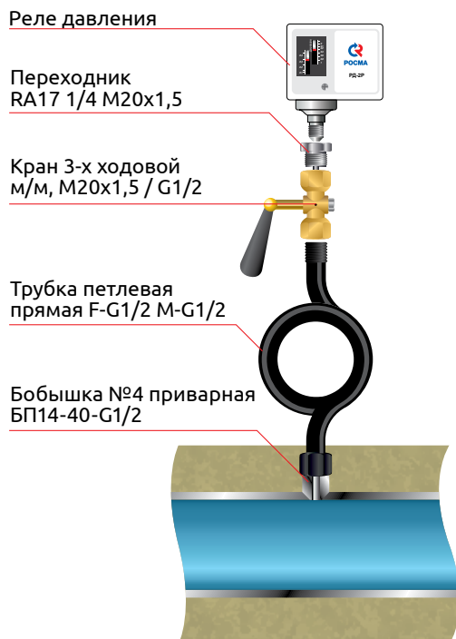
Установка на горизонтальном участке трубопровода
