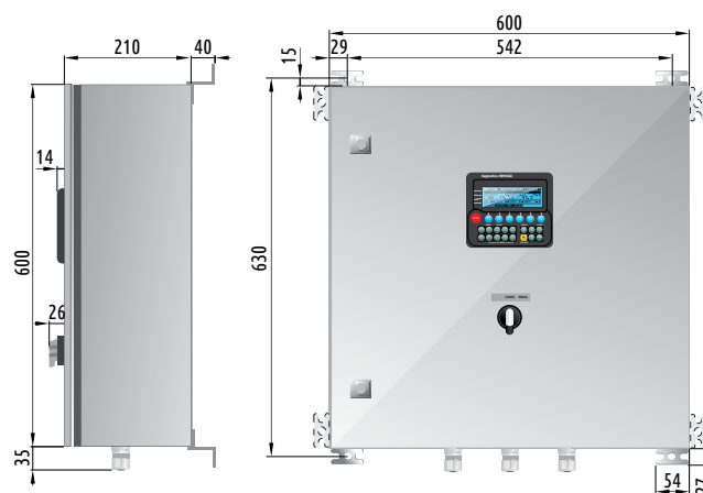
Шкаф управления КОНТУР-С2/3/4 600×600×210 мм
