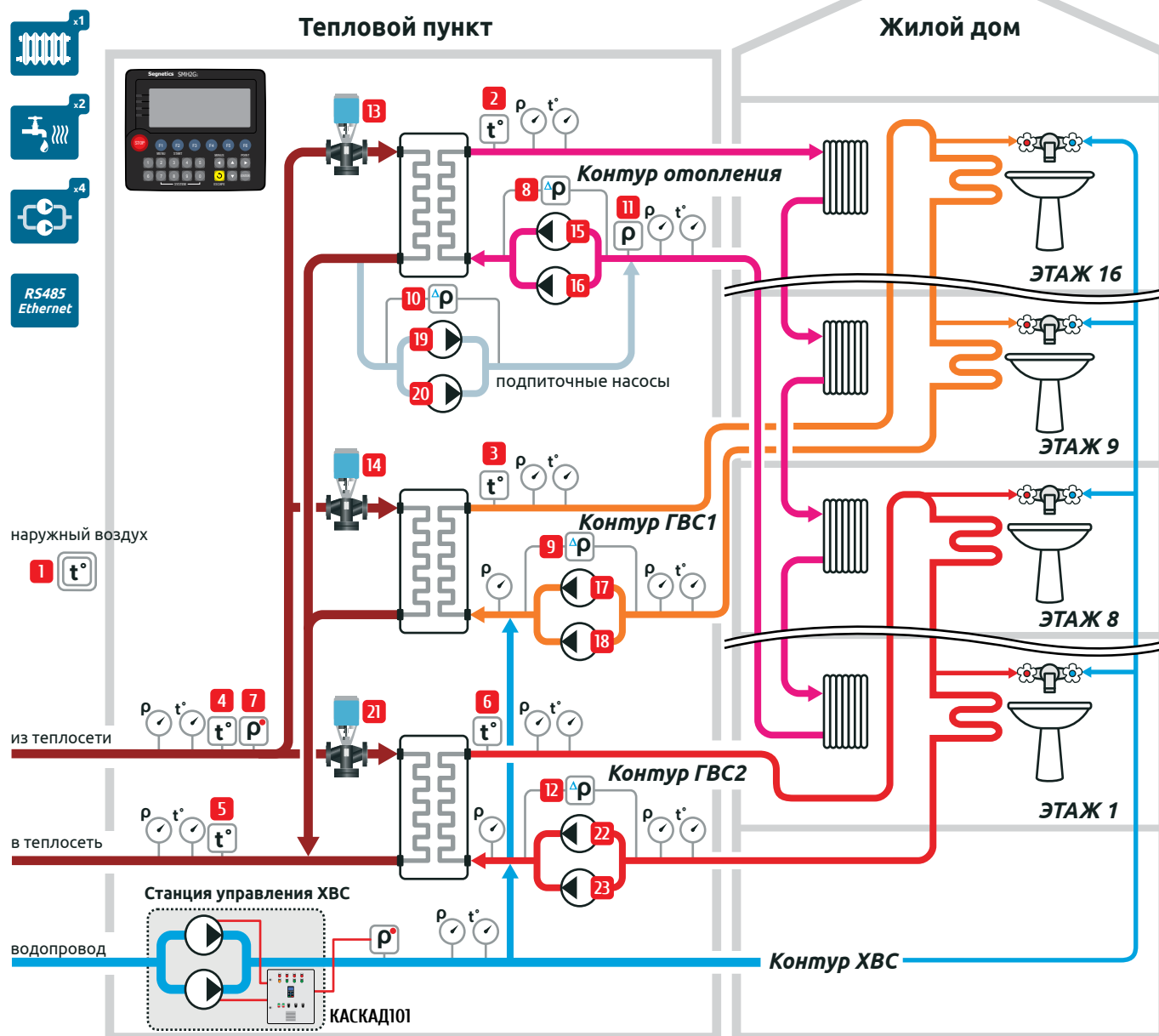
Схема 2 - Типовой ИТП, 1 контур отопления, 2 контура ГВС
