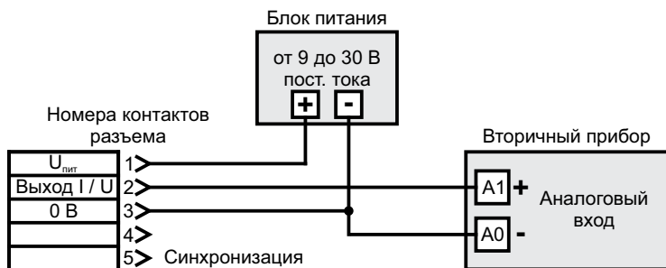
Рисунок 8 – Схема подключения срт+.../IU/TC
