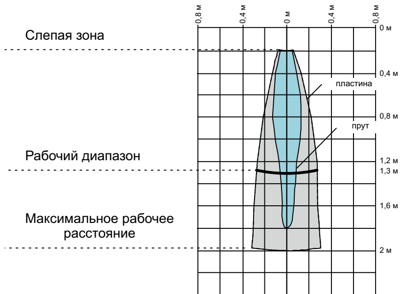
Рисунок 36 – Зона распространения ультразвуковой волны датчика \text{cm}+130/...
