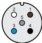
Рисунок 5 – Расположение контактов разъема со стороны датчика
