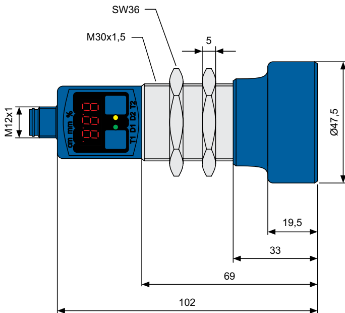
Рисунок 2 – Габаритные размеры cm+340/...
