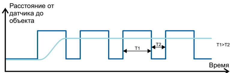
Рисунок 24 — Алгоритм работы датчика с усредняющим фильтром
