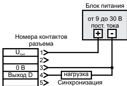
Рисунок 6 – Схема подключения сгт+.../D/TC
