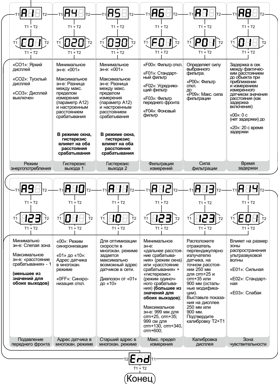
Рисунок 15 – Расширенные настройки параметров датчика см+.../DD/TC
