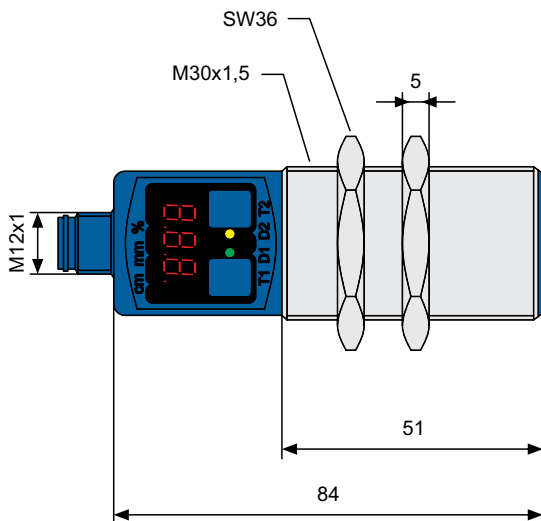
Рисунок 1 – Габаритные размеры cm+25/... , cm+35/... , cm+130/...
