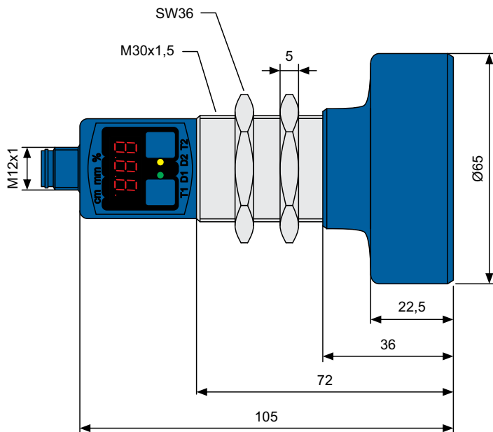
Рисунок 3 – Габаритные размеры стм+600/...
