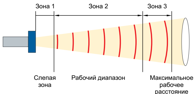
Рисунок 29 – Зоны, соответствующие расстояниям, на которых следует располагать объект
