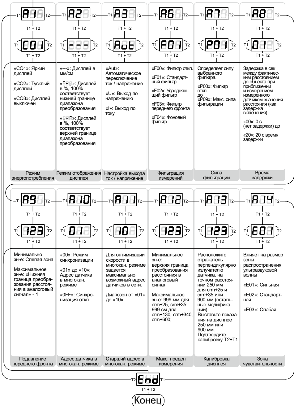
Рисунок 18 – Расширенные настройки параметров датчика стм+.../IU/TC
