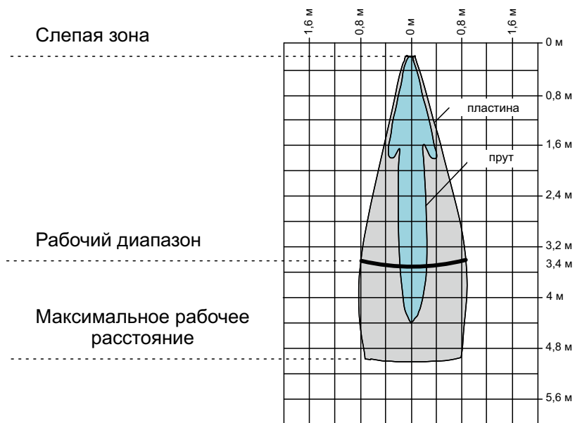
Рисунок 37 – Зона распространения ультразвуковой волны датчика \text{cm}+340/...
