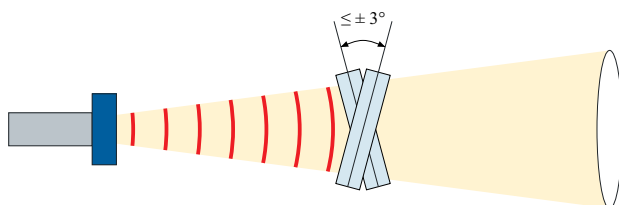
Рисунок 30 – Допустимый угол монтажа при работе с гладкими поверхностями
