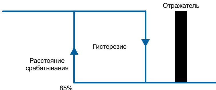
Рисунок 22 – Диаграмма работы дискретного выхода в режиме работы с отражателем
