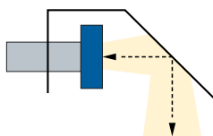
Рисунок 33 – Перенаправление ультразвуковой волны с помощью отражателя
