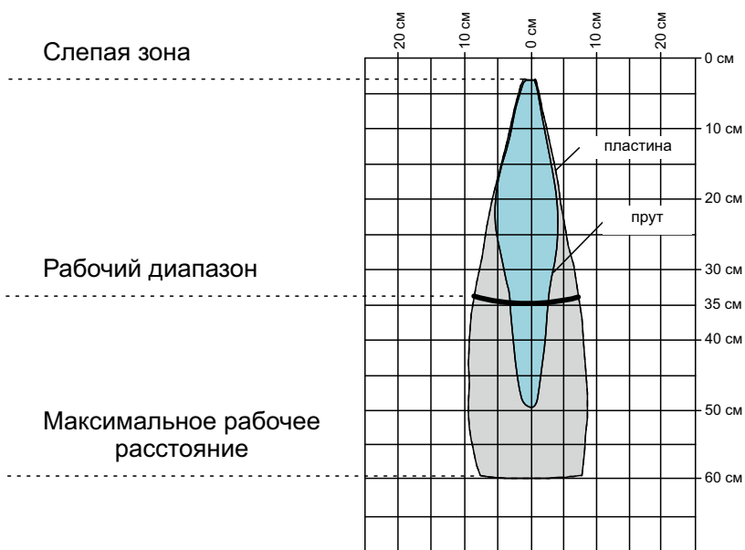
Рисунок 35 – Зона распространения ультразвуковой волны датчика cm+35/...
