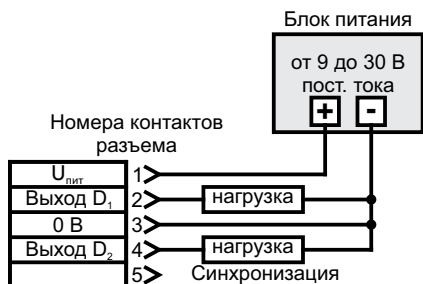
Рисунок 7 – Схема подключения срт+.../DD/TC
