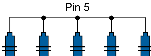
Рисунок 28 – Работа датчиков в режиме синхронизации
