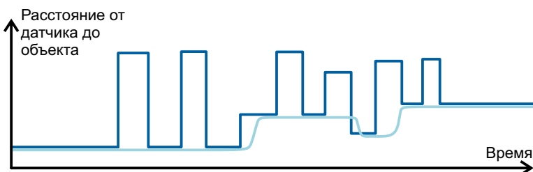
Рисунок 26 – Алгоритм работы датчика с фоновым фильтром
