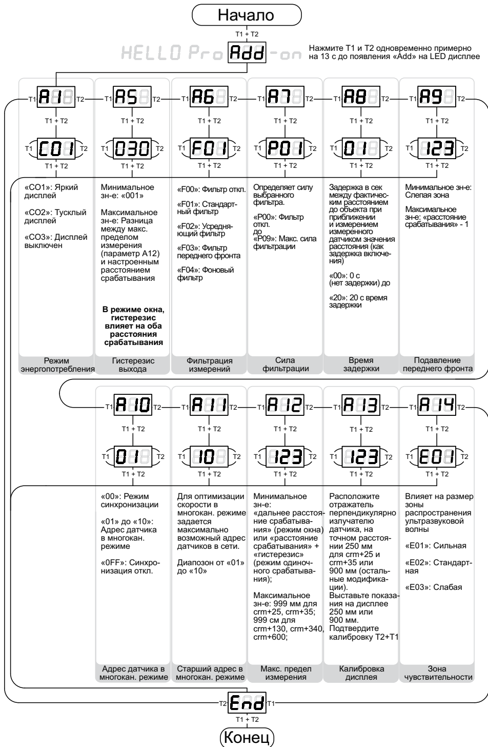
Рисунок 11 – Расширенные настройки параметров датчика cm+.../D/TC
