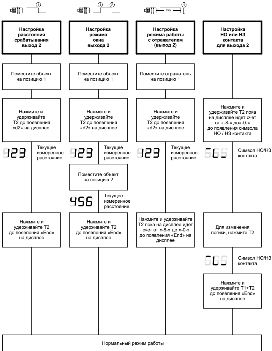
Рисунок 14 – Задание параметров с помощью процедуры «обучения» (дискретный выход 2) для датчика срт+.../DD/TC
