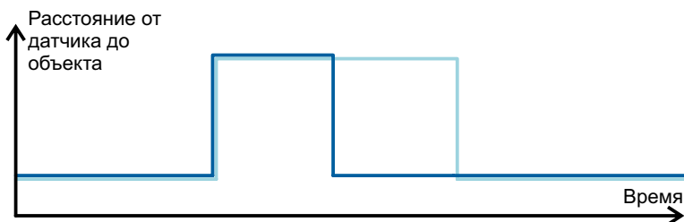
Рисунок 23 — Алгоритм работы датчика со стандартным фильтром
