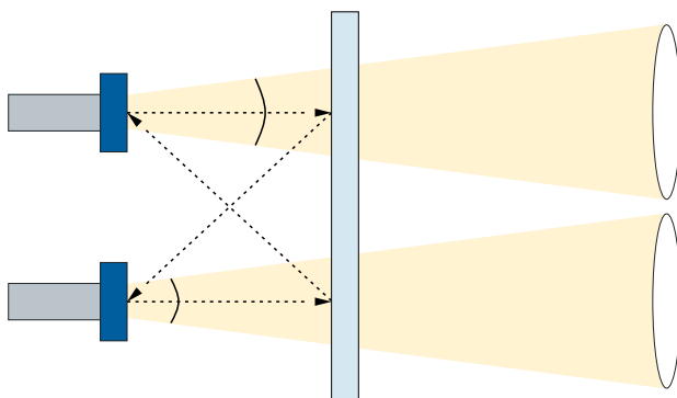
Рисунок 27 – Взаимное влияние датчиков при работе рядом друг с другом
