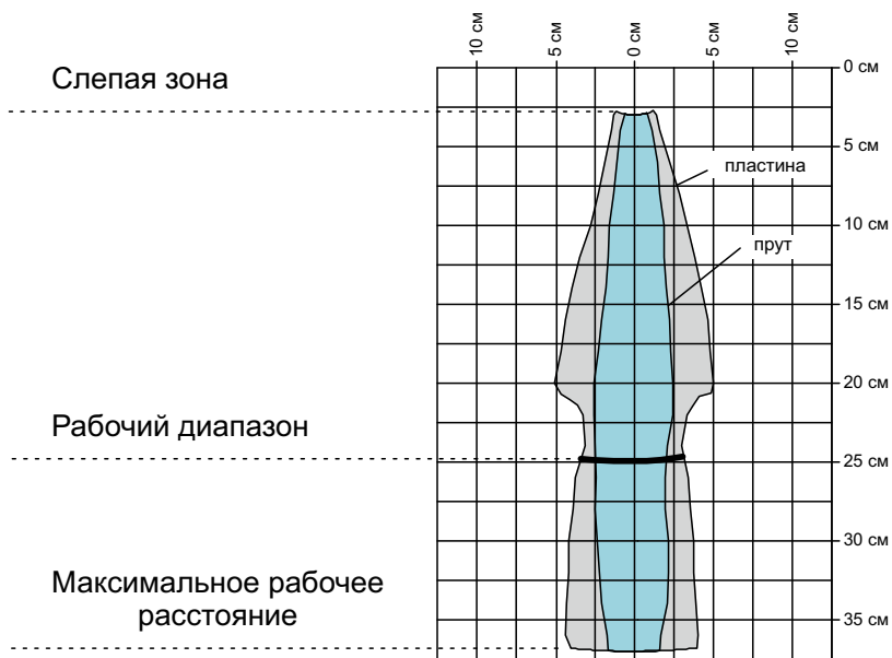
Рисунок 34 – Зона распространения ультразвуковой волны датчика cm+25/...
