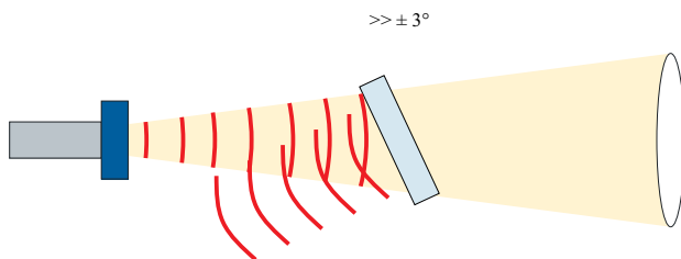
Рисунок 31 – Отражение ультразвукового импульса под углом
