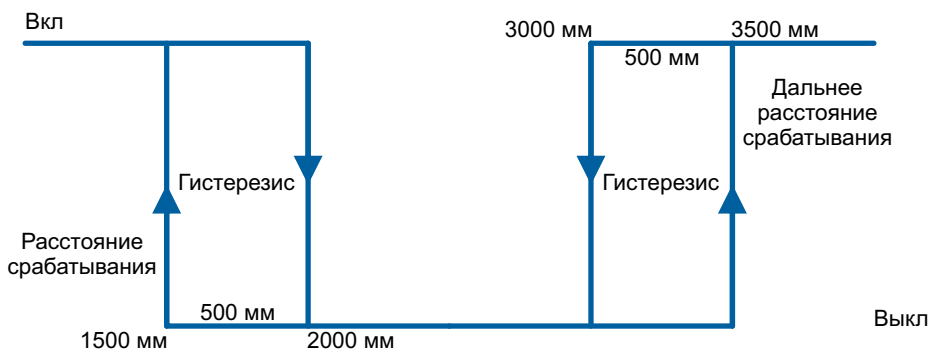
Рисунок 21 – Диаграмма работы дискретного выхода в режиме окна
