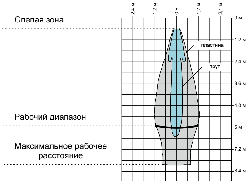
Рисунок 38 – Зона распространения ультразвуковой волны датчика см+600/...
