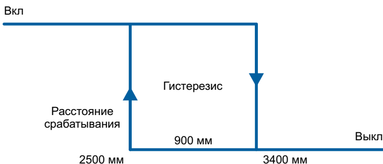
Рисунок 20 – Диаграмма работы дискретного выхода в режиме одиночного срабатывания
