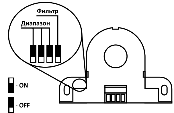
Рисунок 6 – Расположение DIP переключателей
